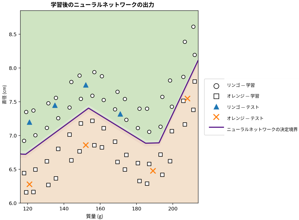
図 7: ニューラルネットワークの学習後に得られた Python の出力。合成データ集合には、質量-直径平面の広い領域に分布する 64 個の学習例と、説明用テストとして別に確保した 8 個の例が含まれる。強調された曲線は \hat{y} = 0.5 の等値線であり、学習された決定境界を表す。色付きの領域はネットワークが予測するクラスを示す。円は学習用リンゴ、四角は学習用オレンジ、三角はテスト用リンゴ、× 印はテスト用オレンジを表す。
