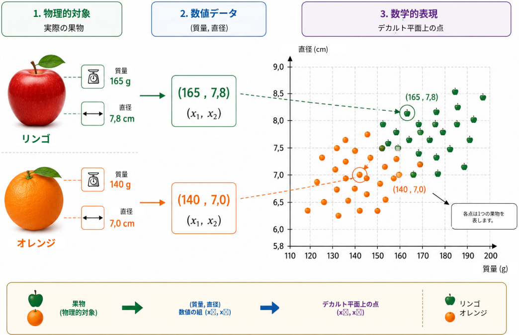
図 1: 物理的観察から数学的モデル化へ。各果物はまず、質量と直径という二つの測定可能な量によって記述され、その後、順序対 (x_1, x_2) で表される。質量-直径平面では各観測が一つの点となるため、リンゴとオレンジの識別は二つのクラスを分離する幾何学的問題として捉え直すことができる。
