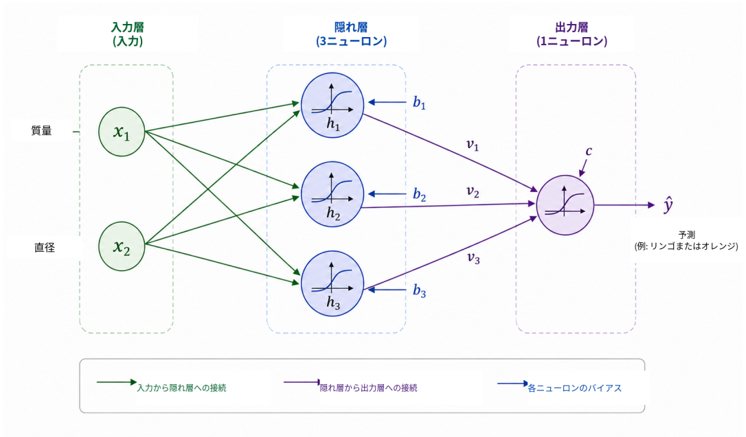
図 5: ニューラルネットワークの計算を導入するための教育的な 2-3-1 構成。二つの入力、すなわち質量と直径が、隠れ層の三つのニューロンへ入力される。そこで得られた活性 h_1, h_2, h_3 を出力ニューロンが組み合わせ、予測 \hat{y} を生成する。すべての接続には調整可能な重みがあり、各ニューロンにはバイアスがある。
