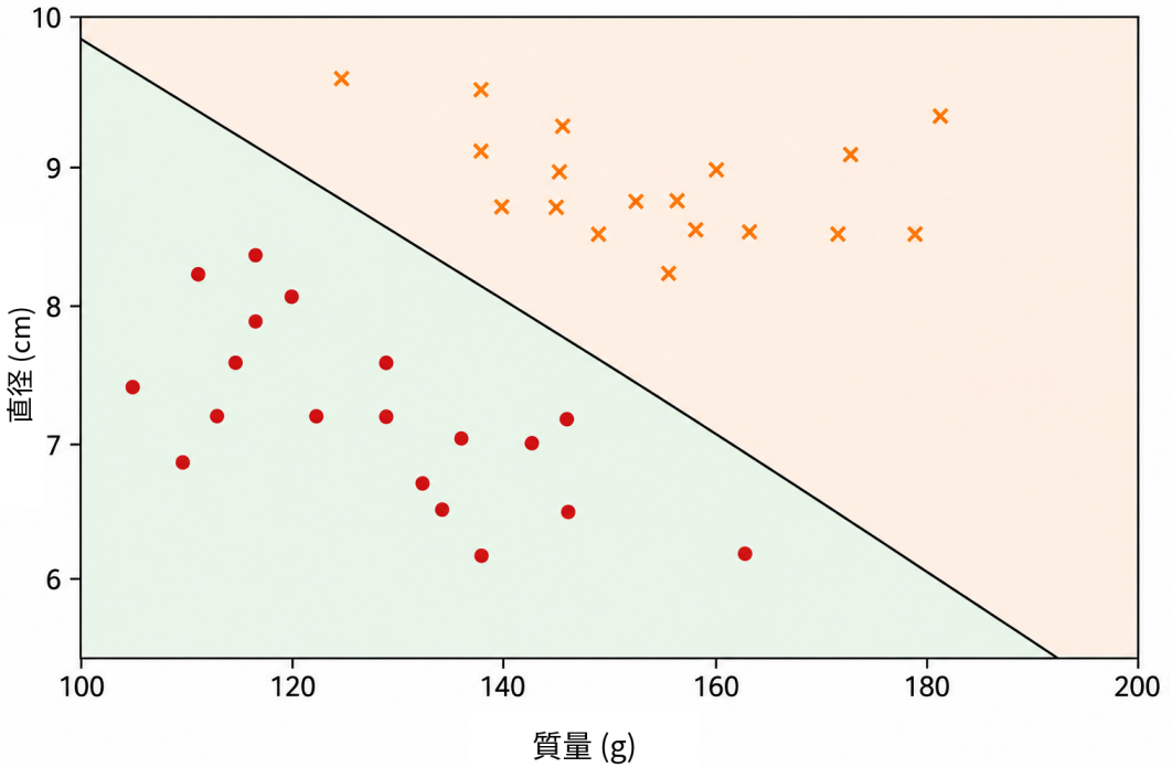
図 2: 質量-直径平面における線形分類器の例。直線は決定境界として働き，一方の半平面にある点には一つのクラスが，他方の半平面にある点には別のクラスが割り当てられる。したがって判断は，点が直線のどちら側にあるかで決まる。
