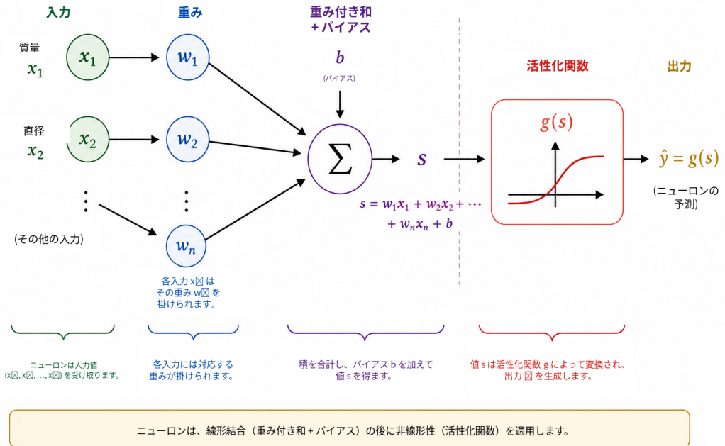
図 3: 人工ニューロンの模式的な動作。各入力 x_i に重み w_i を掛け、それらの積をバイアス b と加えてスコア s を得る。次に活性化関数 g がこのスコアを出力 \hat{y} = g(s) に変換する。この出力は中間量としても最終予測としても利用できる。
