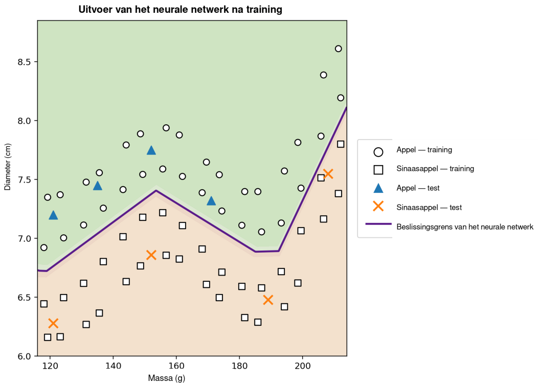
Figuur 7: Python-uitvoer na training van het neurale netwerk. De synthetische gegevensverzameling bevat 64 trainingsvoorbeelden verspreid over een groot gebied van het massa–diameter vlak en acht extra voorbeelden die zijn gereserveerd voor een illustratieve test. De gemarkeerde kromme is het niveau \hat{y} = 0.5 en stelt de geleerde beslissingsgrens voor; de gearceerde gebieden geven de door het netwerk voorspelde klassen aan. Cirkels stellen trainingsappels voor, vierkanten trainingssinaasappels, driehoeken testappels en kruisen testsinaasappels.
