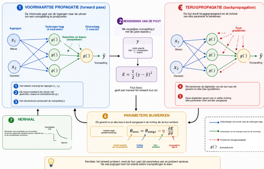
Figuur 6: Basistrainingscyclus van een neuraal netwerk. De forward pass zet de ingangen om in een voorspelling; de verliesfunctie meet het verschil tussen voorspelling en doelwaarde; terugpropagatie berekent gradiënten met de kettingregel; en gradiëntafdeling gebruikt die gradiënten om gewichten en biases bij te werken. Het herhalen van deze cyclus gedurende veel epochs noemen we leren.
