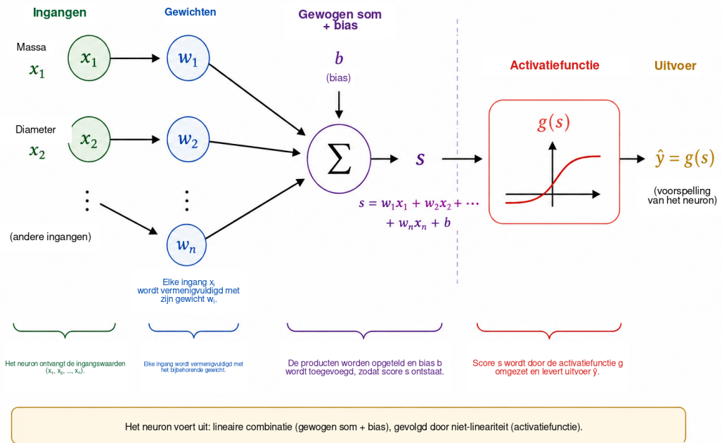
Figuur 3: Schematische werking van een kunstmatig neuron. Elke ingang x_i wordt vermenigvuldigd met een gewicht w_i ; de producten worden samen met bias b opgeteld om score s te produceren. De activatiefunctie g zet deze score vervolgens om in de uitvoer \hat{y} = g(s) , die als tussengrootheid of als uiteindelijke voorspelling kan worden gebruikt.
