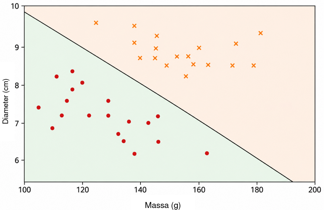
Figuur 2: Voorbeeld van een lineaire classifieer in het massa–diameter vlak. De rechte lijn fungeert als beslissingsgrens: punten in het ene halfvlak krijgen de ene klasse, terwijl punten in het tegenoverliggende halfvlak de andere klasse krijgen. De beslissing hangt dus uitsluitend af van de kant van de rechte waarop het punt ligt.
