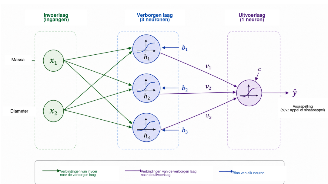
Figuur 5: Didactische 2–3–1-architectuur om de berekening in een neuraal netwerk te introduceren. De twee ingangen — massa en diameter — voeden drie neuronen in de verborgen laag. Hun activiteiten h_1, h_2, h_3 worden vervolgens door het uitvoerneuron gecombineerd om de voorspelling \hat{y} te produceren. Elke verbinding heeft een aanpasbaar gewicht en elk neuron heeft een bias.
