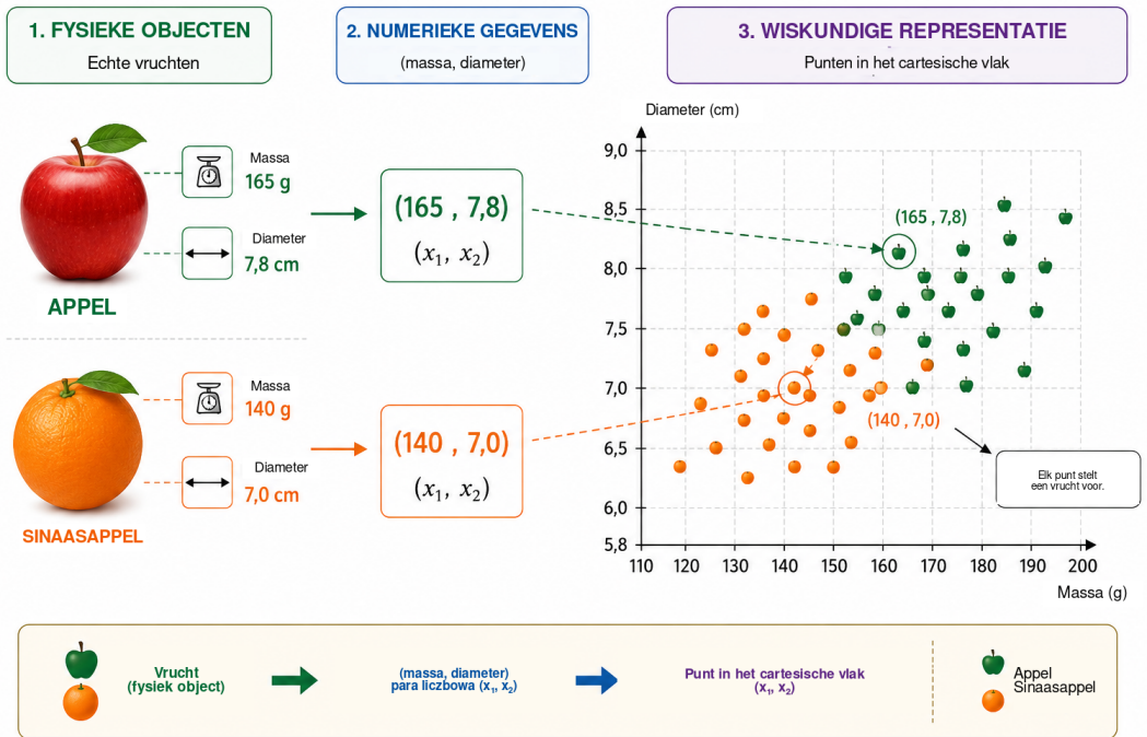
Figuur 1: Van fysieke waarneming naar wiskundige modellering. Elke vrucht wordt eerst beschreven door twee meetbare grootheden — massa en diameter — en vervolgens voorgesteld door het geordende paar (x_1, x_2) . In het massa–diameter vlak wordt elke waarneming een punt, zodat het onderscheiden van appels en sinaasappels kan worden geherinterpreteerd als een meetkundig probleem van het scheiden van twee klassen.
