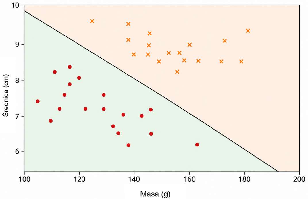
Rysunek 2: Przykład klasyfikatora liniowego na płaszczyźnie masa–średnica. Prosta pełni rolę granicy decyzyjnej: punkty w jednej półpłaszczyźnie otrzymują jedną klasę, a punkty w przeciwnej półpłaszczyźnie drugą. Decyzja zależy zatem wyłącznie od tego, po której stronie prostej znajduje się punkt.
