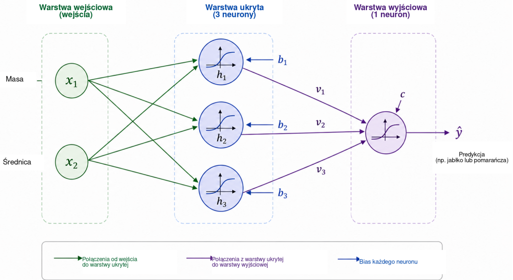
Rysunek 5: Dydaktyczna architektura 2–3–1 użyta do wprowadzenia obliczeń w sieci neuronowej. Dwa wejścia — masa i średnica — zasilają trzy neurony warstwy ukrytej. Ich aktywacje h_1, h_2, h_3 są następnie łączone przez neuron wyjściowy, który tworzy predykcję \hat{y} . Każde połączenie ma regulowaną wagę, a każdy neuron ma bias.
