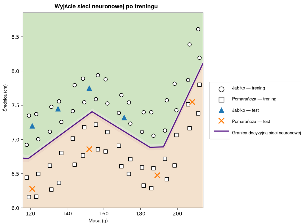
Rysunek 7: Wynik programu w Pythonie po treningu sieci neuronowej. Syntetyczny zbiór danych zawiera 64 przykłady treningowe rozmieszczone na szerokim obszarze płaszczyzny masa–średnica oraz osiem dodatkowych przykładów przeznaczonych do ilustracyjnego testu. Wyróżniona krzywa jest poziomnicą \hat{y} = 0.5 i reprezentuje nauczoną granicę decyzyjną; zacieniowane obszary wskazują klasy przewidywane przez sieć. Okręgi oznaczają jabłka treningowe, kwadraty pomarańcze treningowe, trójkąty jabłka testowe, a krzyżyki pomarańcze testowe.
