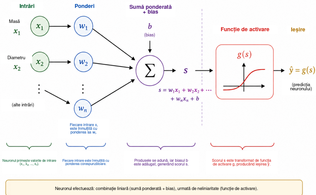
Figura 3: Schema de funcționare a unui neuron artificial. Fiecare intrare x_i este înmulțită cu o pondere w_i ; produsele sunt adunate la biasul b pentru a produce scorul s . Funcția de activare g transformă apoi acest scor în ieșirea \hat{y} = g(s) , care poate fi utilizată ca mărime intermediară sau ca predicție finală.
