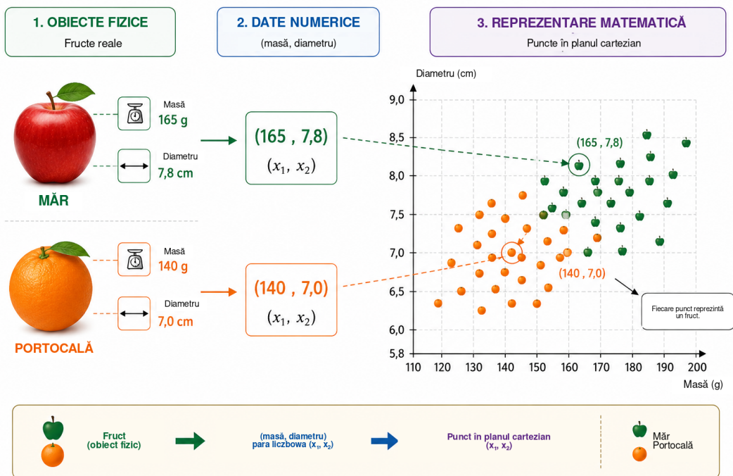
Figura 1: De la observația fizică la modelarea matematică. Fiecare fruct este descris mai întâi prin două mărimi măsurabile — masa și diametrul — și este apoi reprezentat prin perechea ordonată (x_1, x_2) . În planul masă–diametru, fiecare observație devine un punct, astfel încât distingerea merelor de portocale poate fi reinterpretată ca o problemă geometrică de separare a două clase.
