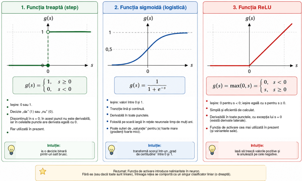
Figura 4: Comparație între trei funcții de activare utilizate frecvent în prezentările introductive ale rețelelor neuronale. Funcția treaptă ia o decizie bruscă; sigmoidea oferă o tranziție netedă între 0 și 1; iar ReLU suprimă intrările negative și le păstrează pe cele pozitive. Activările neliniare împiedică o succesiune de straturi să se reducă la o singură transformare afină.
