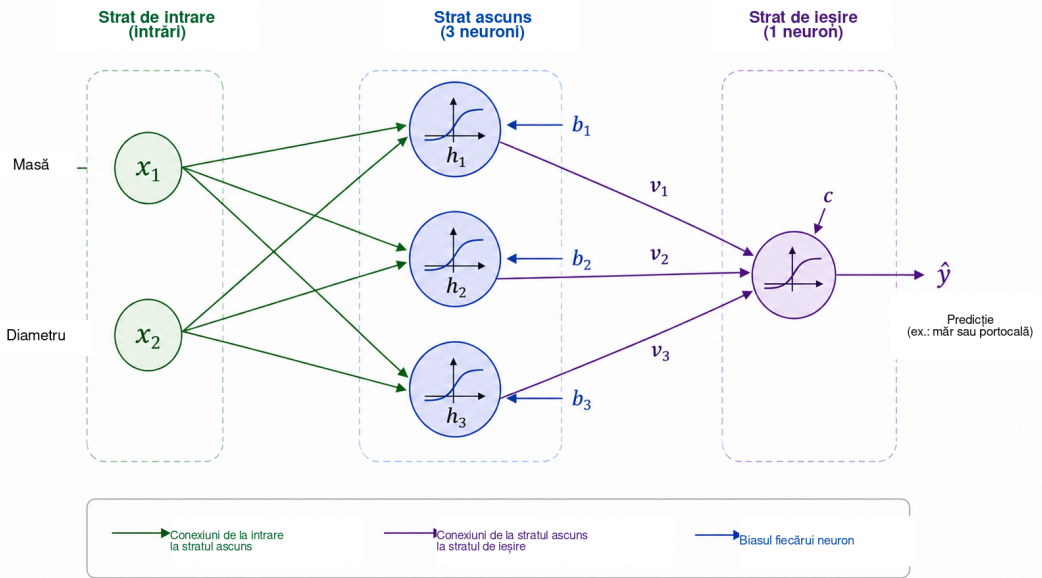
Figura 5: Arhitectură pedagogică 2–3–1 utilizată pentru introducerea calculului într-o rețea neuronală. Cele două intrări — masa și diametrul — alimentează trei neuroni din stratul ascuns. Activările lor h_1, h_2, h_3 sunt apoi combinate de neuronul de ieșire pentru a produce predicția \hat{y} . Fiecare conexiune are o pondere ajustabilă, iar fiecare neuron are un bias.
