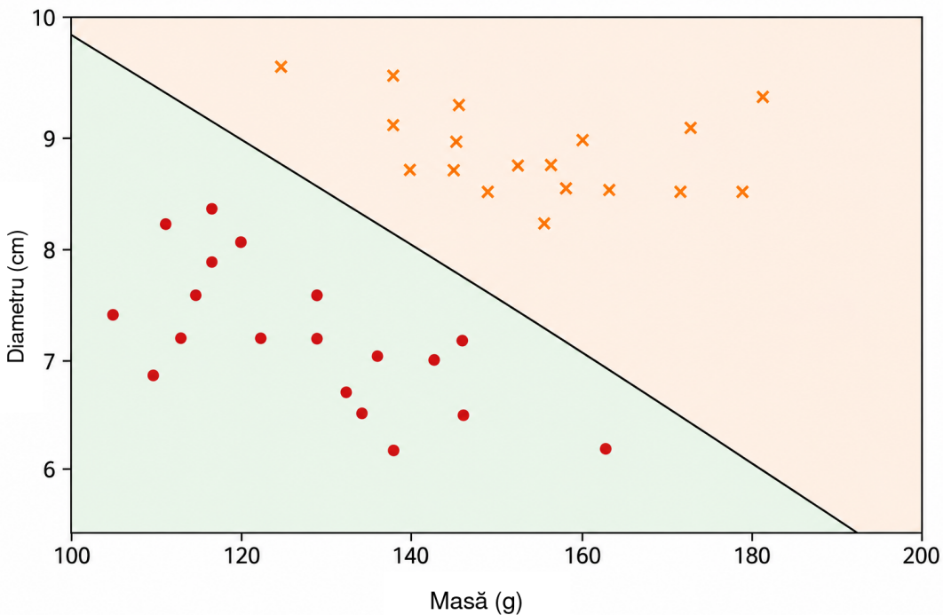
Figura 2: Exemplu de clasificator linear în planul masă–diametru. Dreapta joacă rolul unei frontiere de decizie: punctele dintr-un semiplan primesc o clasă, iar punctele din semiplanul opus primesc cealaltă clasă. Decizia depinde, așadar, numai de partea drepte în care se află punctul.
