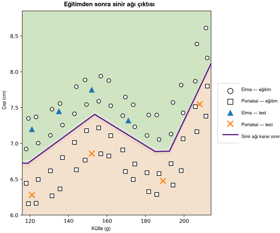
Şekil 7: Sinir ağının eğitiminden sonra elde edilen Python çıktısı. Sentetik veri kümesi, kütle-çap düzleminin geniş bir bölgesine yayılmış 64 eğitim örneği ve açıklayıcı bir test için ayrılmış sekiz ek örnek içerir. Vurgulanan eğri \hat{y} = 0.5 düzeyidir ve öğrenilen karar sınırını temsil eder; gölgeli bölgeler ağın tahmin ettiği sınıfları gösterir. Daireler eğitim elmaları, kareler eğitim portakalları, üçgenler test elmaları ve çarpılar test portakallarıdır.
