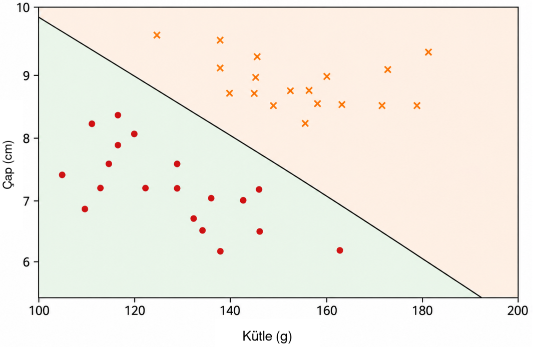
Şekil 2: Kütle-çap düzleminde doğrusal sınıflandırıcı örneği. Doğru bir karar sınırı olarak işlev görür: bir yarı düzlemdeki noktalar bir sınıfa, karşı yarı düzlemdeki noktalar diğer sınıfa atanır. Dolayısıyla karar yalnızca noktanın doğrunun hangi tarafında bulunduğuyla bağlıdır.
