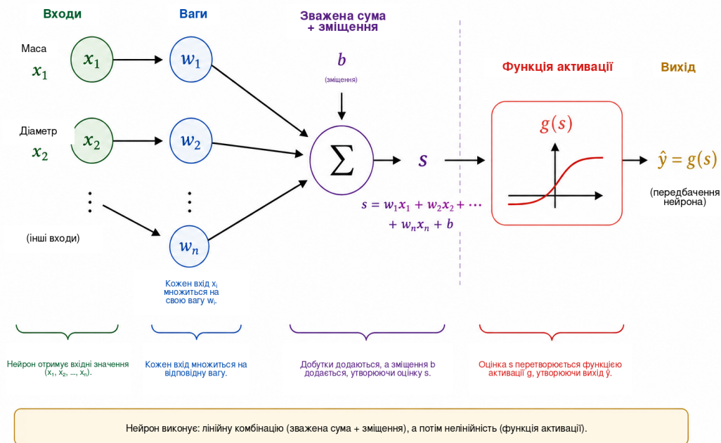
Рис. 3: Схема роботи штучного нейрона. Кожен вхід x_i множиться на вагу w_i ; добутки додаються до зміщення b , утворюючи оцінку s . Потім функція активації g перетворює цю оцінку на вихід \hat{y} = g(s) , який може бути проміжною величиною або кінцевим передбаченням.
