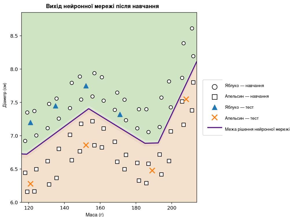
Рис. 7: Вихід Python після навчання нейронної мережі. Синтетичний набір даних містить 64 навчальні приклади, розподілені по широкій області площини “маса–діаметр”, і вісім додаткових прикладів, зарезервованих для ілюстративного тесту. Виділена крива є рівнем \hat{y} = 0.5 і представляє вивчену межу рішення; зафарбовані області показують класи, передбачені мережею. Кола відповідають навчальним яблукам, квадрати — навчальним апельсинам, трикутники — тестовим яблукам, а хрестики — тестовим апельсинам.
