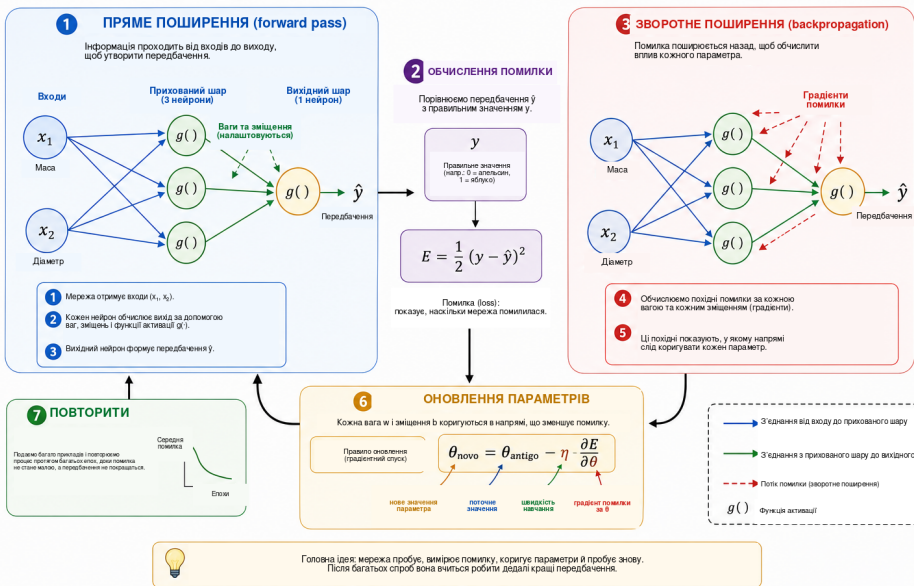
Рис. 6: Базовий цикл навчання нейронної мережі. Прямий прохід перетворює входи на передбачення; функція втрат вимірює невідповідність між передбаченням і ціллю; зворотне поширення обчислює градієнти за правилом ланцюга; градієнтний спуск використовує ці градієнти для оновлення ваг і зміщень. Повторення цього циклу протягом багатьох епох і є навчанням.
