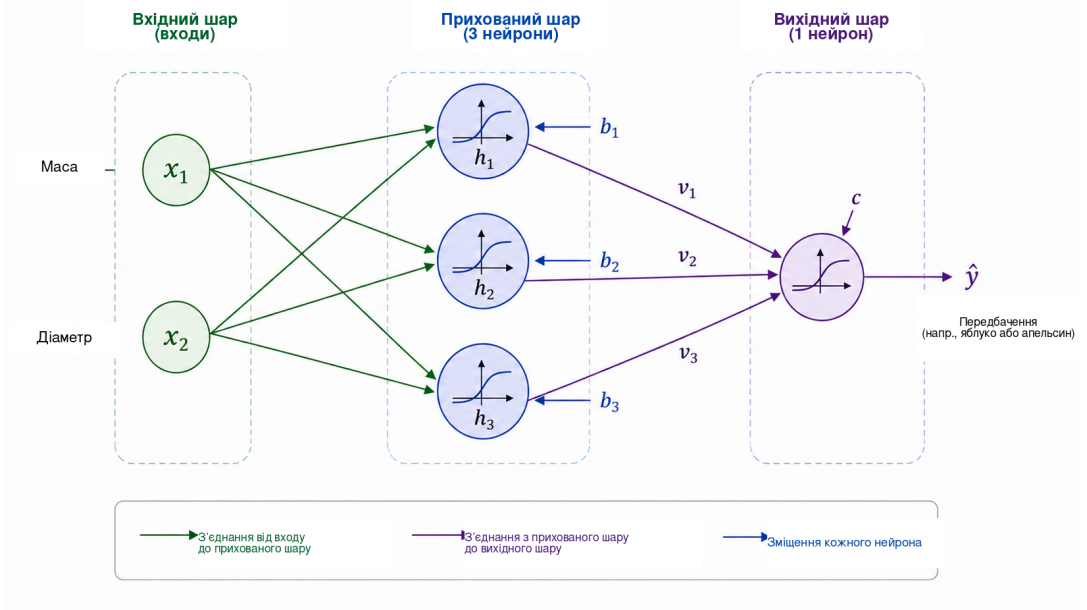
Рис. 5: Дидактична архітектура 2–3–1, використана для введення обчислень у нейронній мережі. Два входи — маса та діаметр — надходять до трьох нейронів прихованого шару. Їхні активації h_1, h_2, h_3 потім комбінуються вихідним нейроном для отримання передбачення \hat{y} . Кожне з'єднання має вагу, що налаштовується, а кожен нейрон — зміщення.
