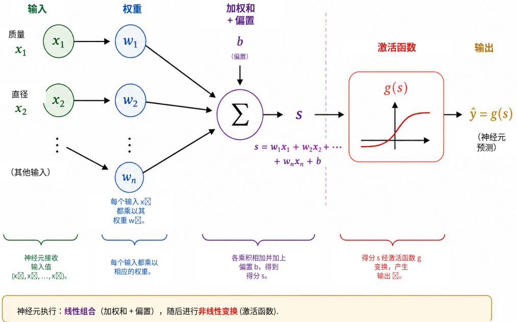
图 3: 人工神经元的示意计算。每个输入 x_i 乘以一个权重 w_i ; 所有乘积与偏置 b 相加, 得到得分 s 。随后激活函数 g 把该得分变换成输出 \hat{y} = g(s) 。这个输出既可以作为网络中的中间量, 也可以作为最终预测。
