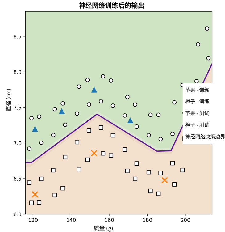
图 7: 神经网络训练后的 Python 输出。合成数据集包含 64 个训练样本，它们分布在质量-直径平面的较大区域中，另外还有八个样本保留用于示意性测试。加粗曲线是等值线 \hat{y} = 0.5 ，表示学得的决策边界；阴影区域表示网络预测的类别。圆圈表示训练苹果，方块表示训练橙子，三角形表示测试苹果，叉号表示测试橙子。
