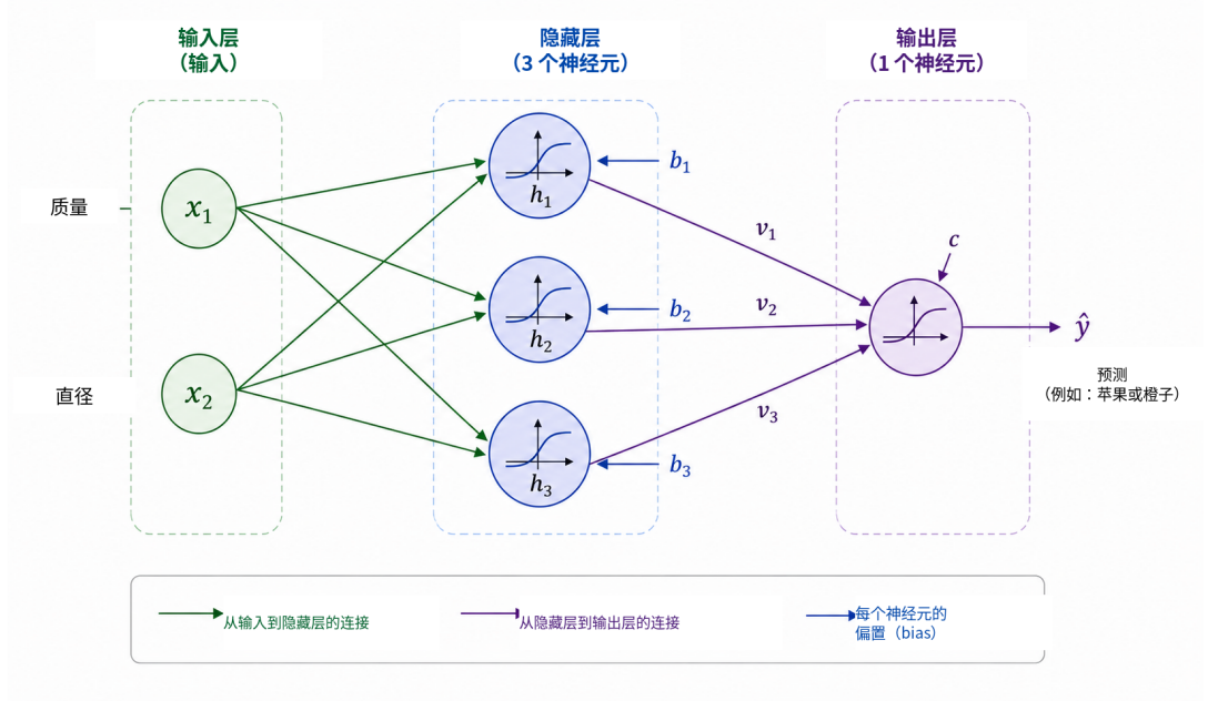
图 5: 用于介绍神经网络计算的教学型 2-3-1 结构。两个输入—质量和直径—连接到隐藏层中的三个神经元。三个激活值 h_1, h_2, h_3 随后由输出神经元组合，得到预测 \hat{y} 。每条连接都具有可调权重，每个神经元都具有偏置。
