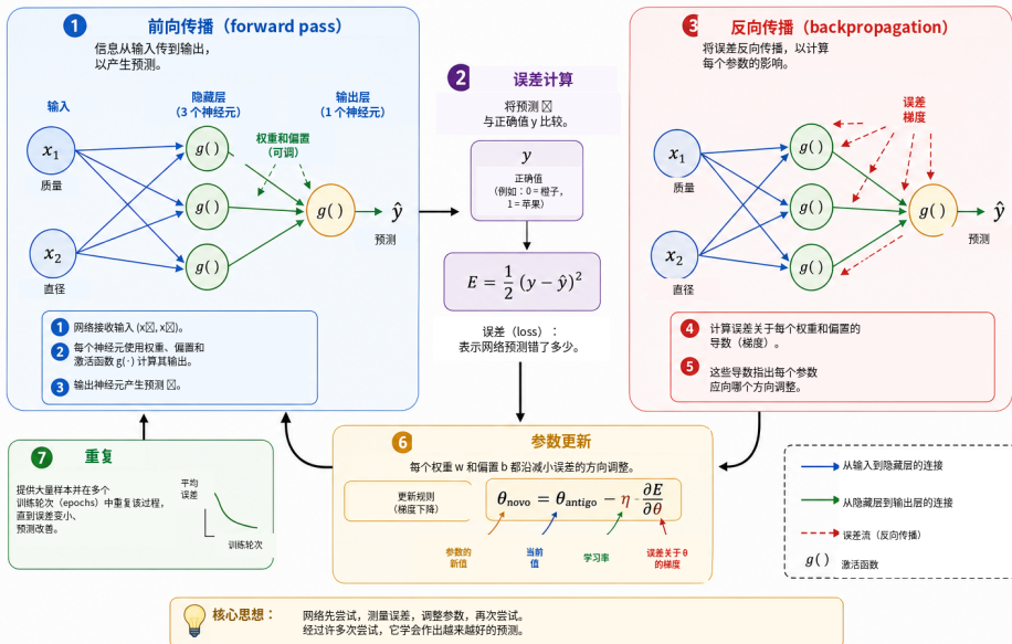
图 6: 神经网络训练的基本循环。前向传播把输入变换成预测；损失函数衡量预测与目标之间的差异；反向传播利用链式法则计算梯度；梯度下降再利用这些梯度更新权重和偏置。经过许多个训练轮次反复执行这个循环，就是所谓的学习。
