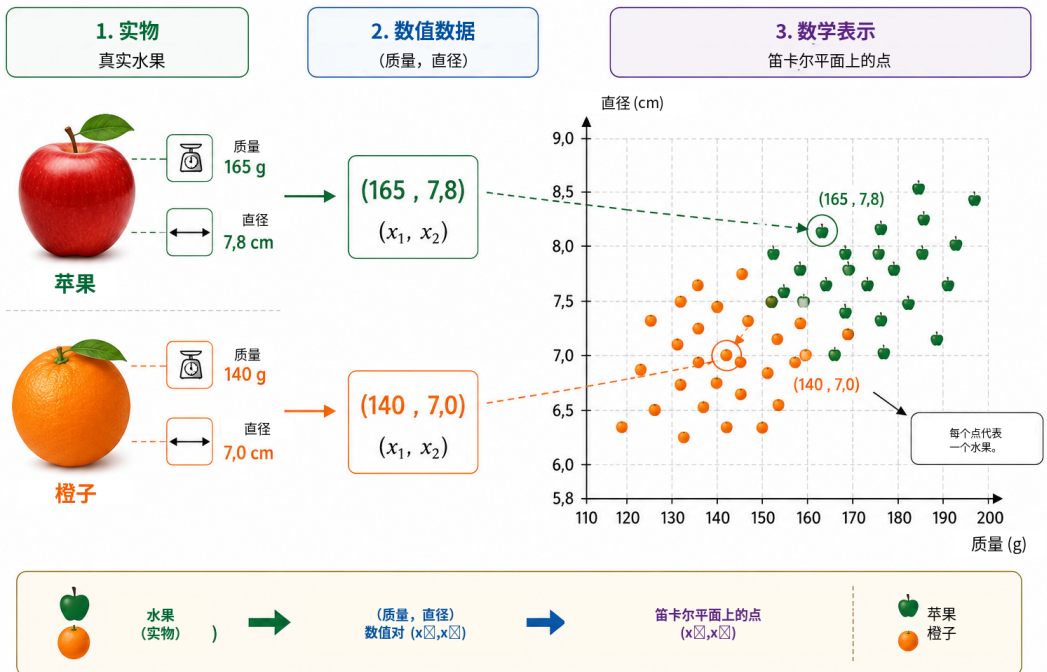
图 1: 从物理观察到数学建模。首先用两个可测量的量—质量和直径—描述每个水果，然后用有序对 (x_1, x_2) 表示它。在质量-直径平面中，每个观测都变成一个点，因此区分苹果和橙子可以重新表述为一个将两类点分开的几何问题。
