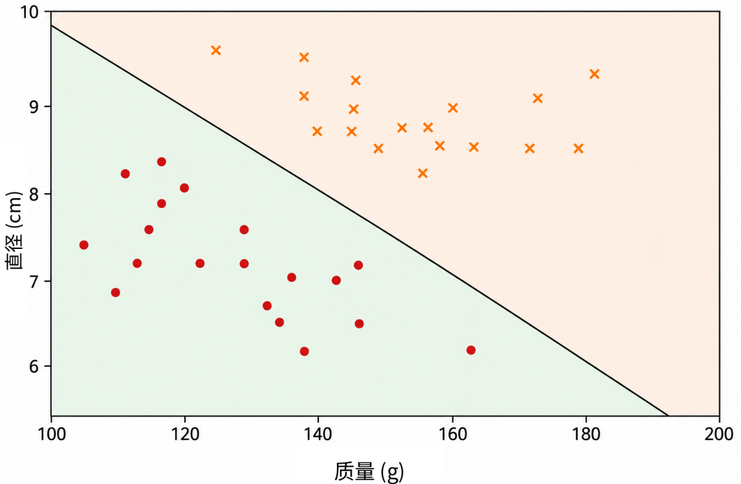
图 2: 质量-直径平面中的线性分类器示例。直线充当决策边界：一个半平面中的点被赋予一类，而另一个半平面中的点被赋予另一类。因此，分类决定只取决于点位于直线的哪一侧。
