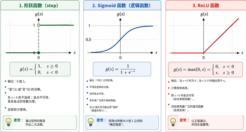
图 4 直观比较了这三种激活函数：阶跃函数的突然跳变、sigmoid 的平滑过渡，以及 ReLU 在零点处斜率的变化。
