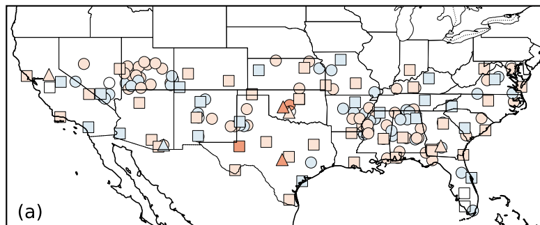
SSA_DA - CNTL
