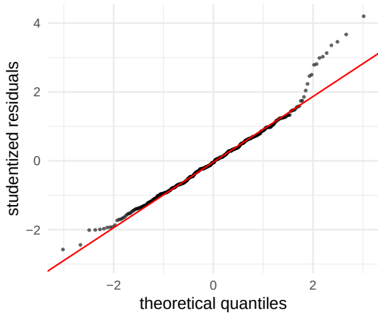
Auto: mpg model
