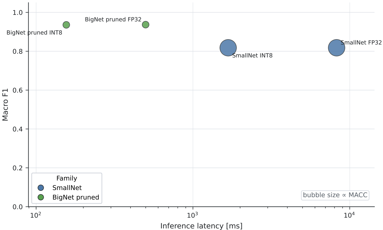
Macro F1 vs Inference Latency
