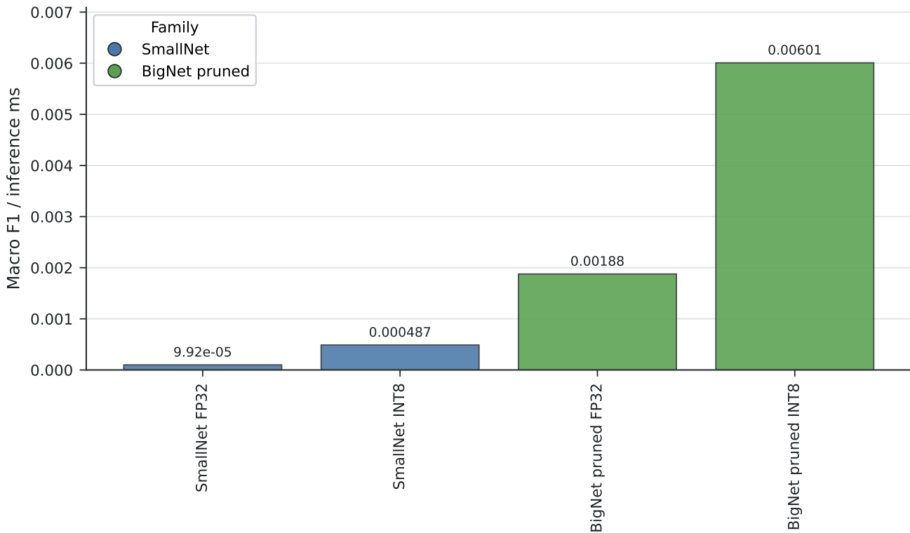
Macro F1 per Inference Millisecond
