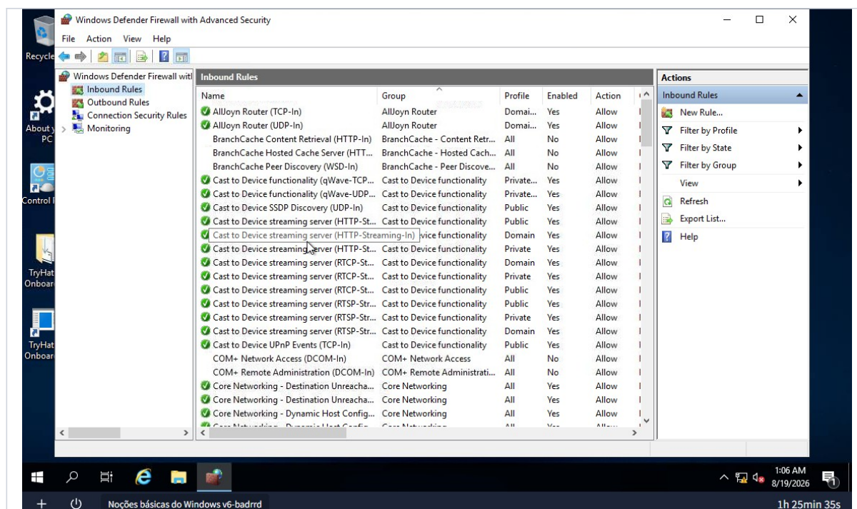
Figura 16 — Lista de regras de entrada do firewall, detalhando nome, grupo, perfil de rede, status e ação de cada regra.
