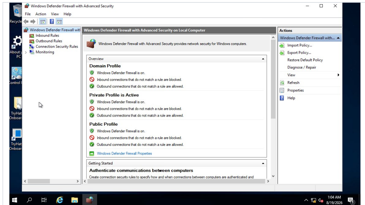
Figura 15 — Visão geral do Firewall do Windows Defender: os três perfis de rede (Domínio, Privado e Público) ativos, com conexões de entrada não correspondentes bloqueadas por padrão.
