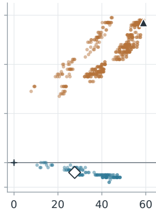
(c) SSP5-8.5 / 2080
