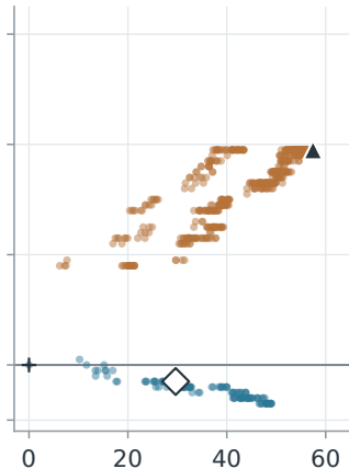
(b) SSP2-4.5 / 2050
