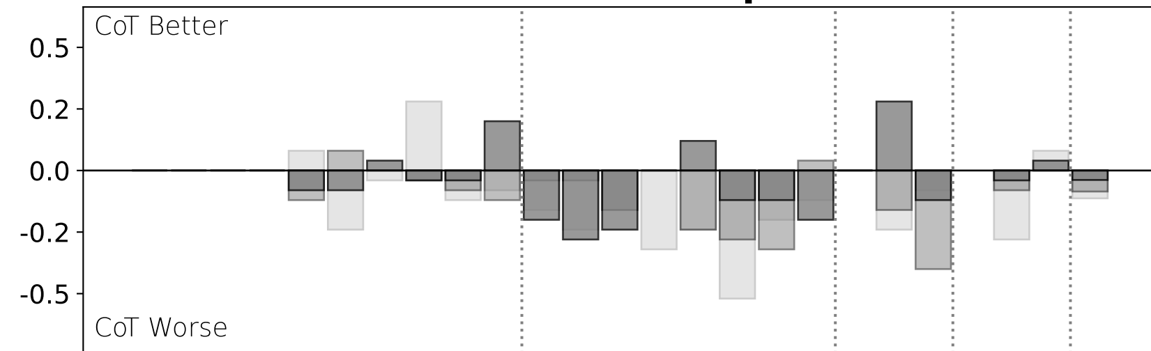
ViPlan-HH: VLM-as-planner
