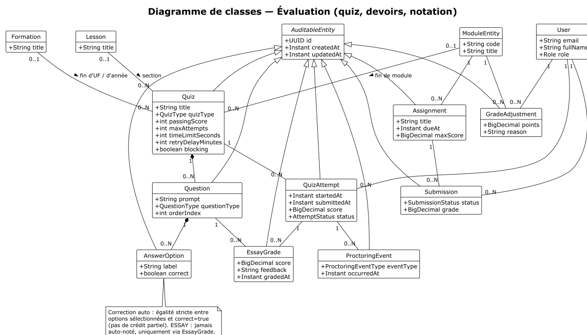
FIGURE 2.4 – Diagramme de classes — évaluation
