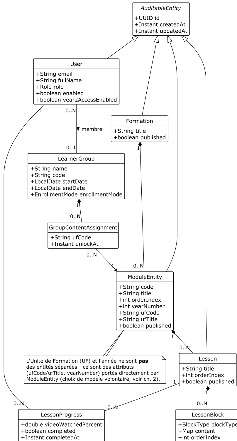
FIGURE 2.3 – Diagramme de classes — structure pédagogique et groupes
