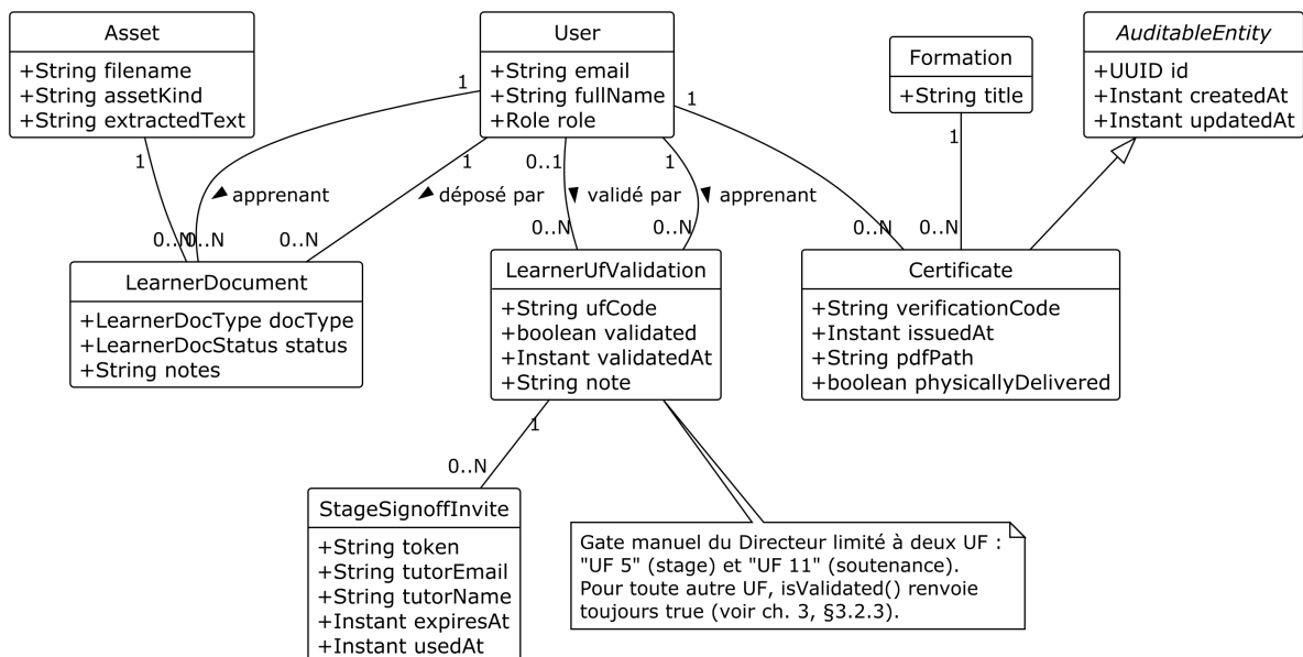
Diagramme de classes — Stage et certification
