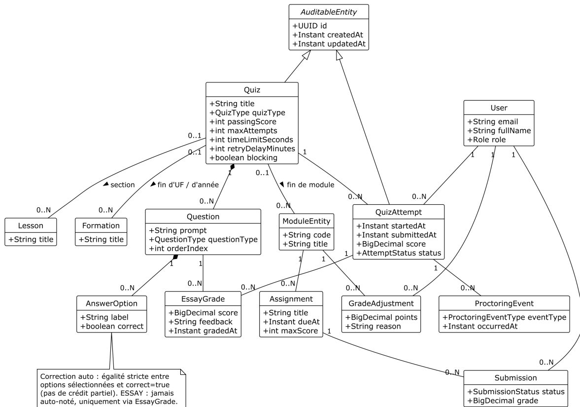
Diagramme de classes — Évaluation (quiz, devoirs, notation)
