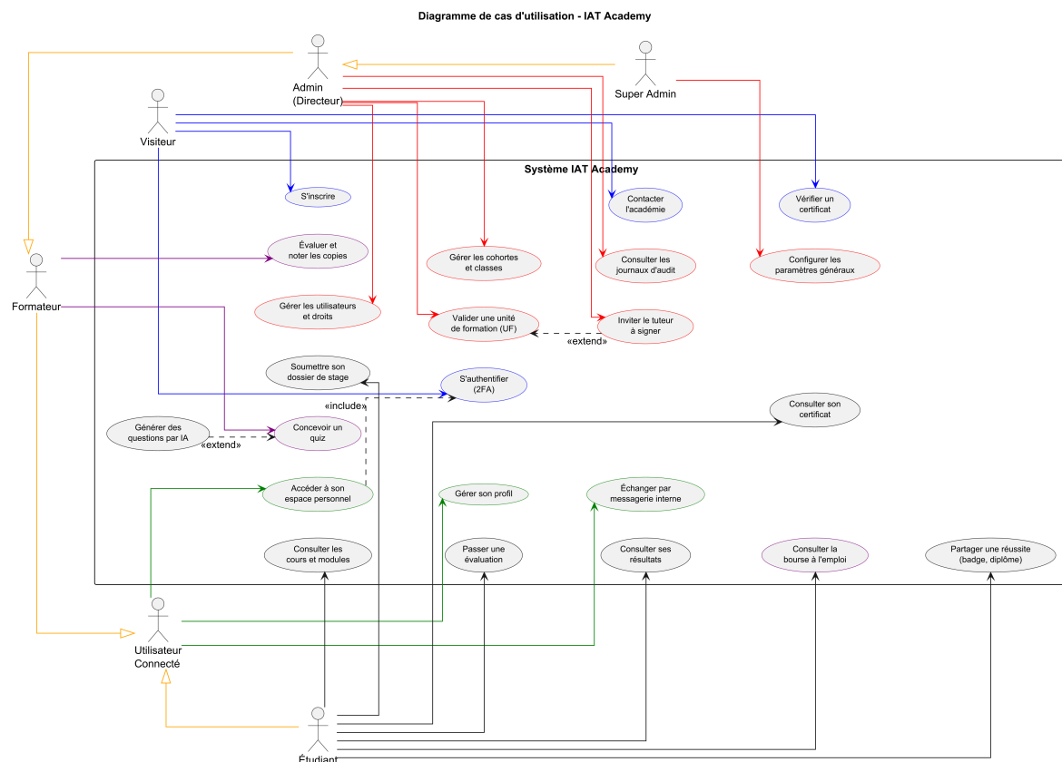
Figure A.2. Diagramme de cas d'utilisation — vue d'ensemble complète (annexe) Descriptif : Version pleine page du diagramme présenté en section 2.4, regroupée ici avec les autres diagrammes UML pour une consultation rapide en soutenance.
