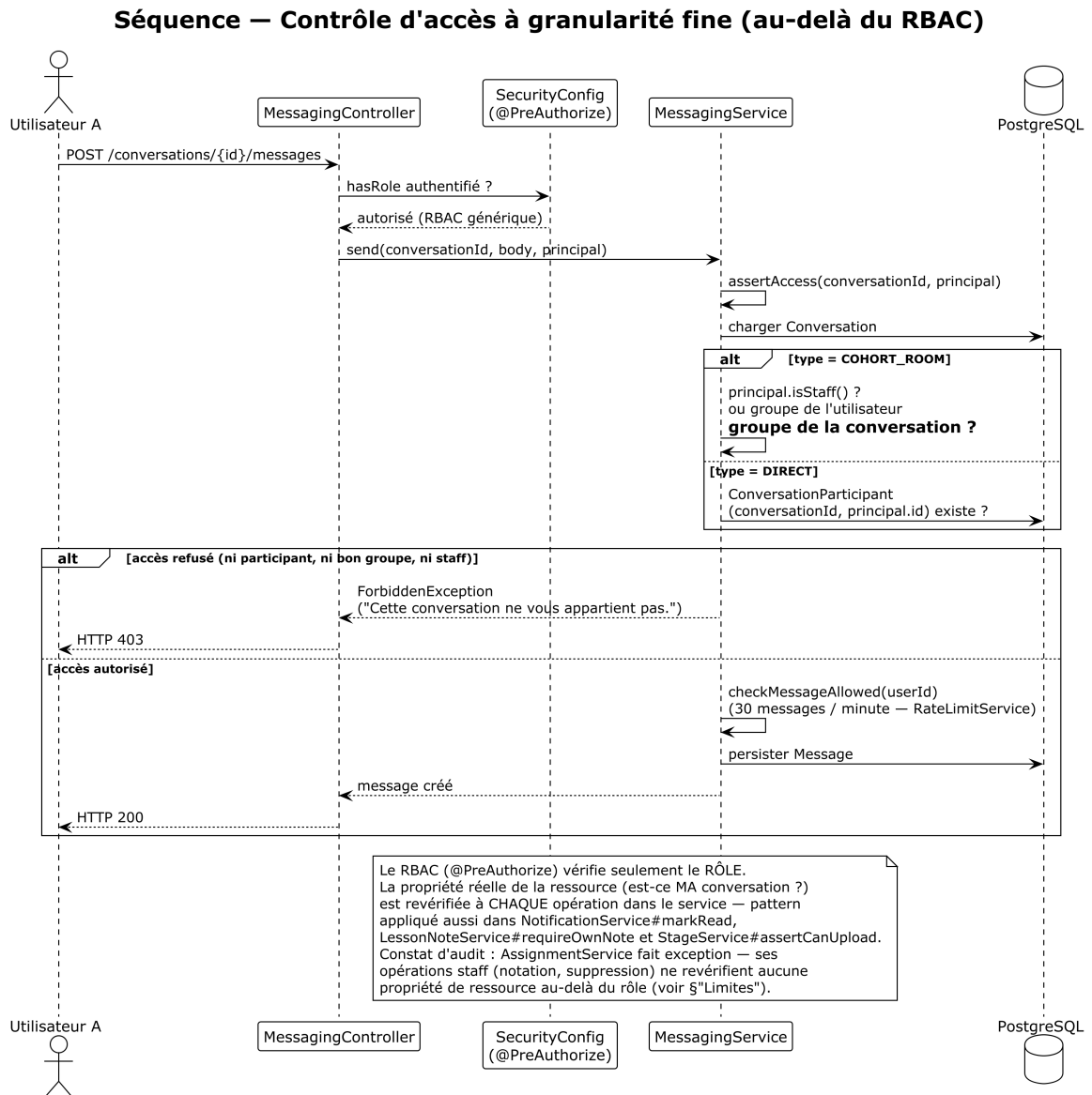
Figure A.6. Contrôle d'accès à granularité fine sur une ressource apprenant (annexe) Descriptif : Correspond au diagramme de séquence de la sous-section consacrée au contrôle d'accès à granularité fine, section 4.3.
