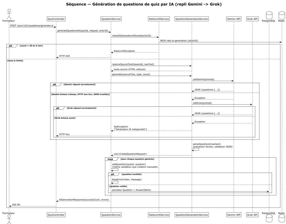
Figure A.3. Génération de questions par IA avec repli Gemini vers Grok (annexe) Descriptif : Correspond à la Figure 4.1, section 4.3.1.
