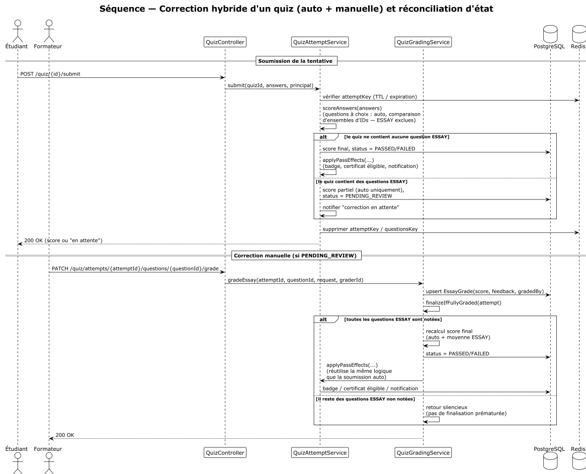
Figure A.4. Correction hybride d'un quiz, automatique puis manuelle (annexe) Descriptif : Correspond au diagramme de séquence de la sous-section consacrée à la correction hybride, section 4.3.
