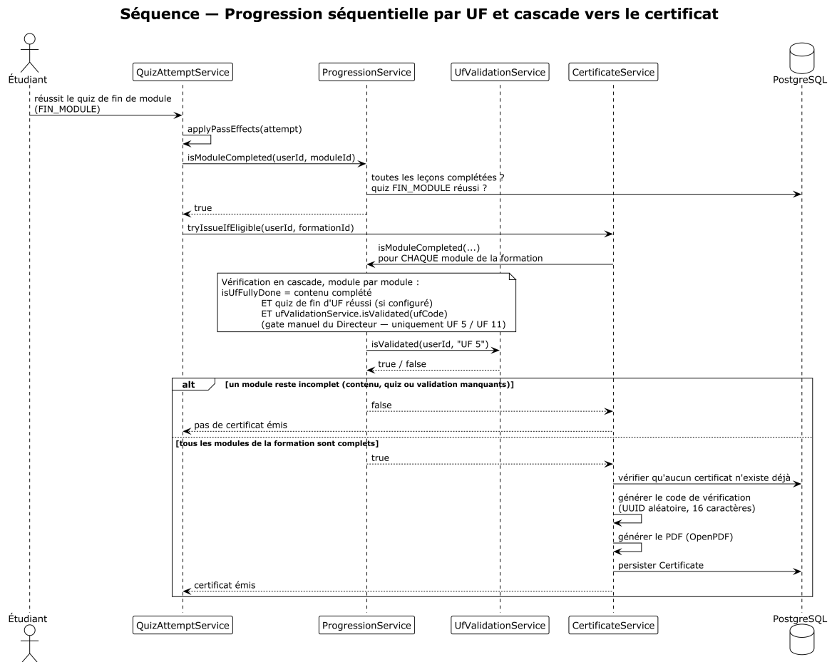
Figure A.5. Progression séquentielle par UF jusqu'au certificat (annexe)
