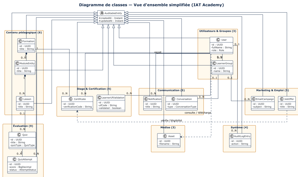
FIGURE 2.2 – Diagramme de classes — vue d'ensemble simplifiée de l'application
