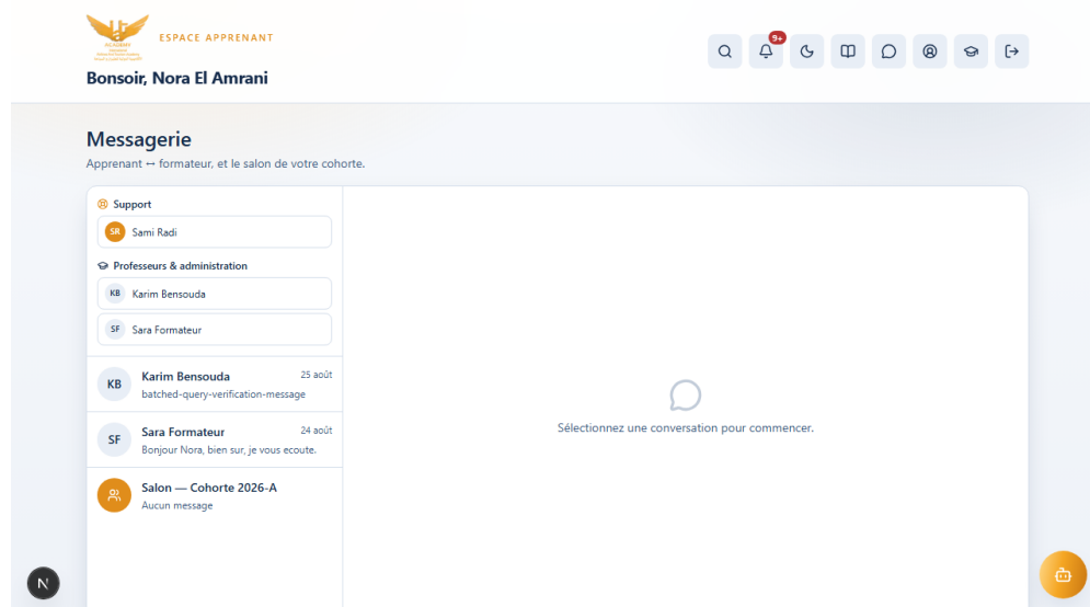
Figure 4.11. Annuaire support épinglé, distinct des professeurs Descriptif : Côté apprenant : le support technique et les professeurs apparaissent comme deux listes de contact séparées, en plus des conversations déjà existantes.
