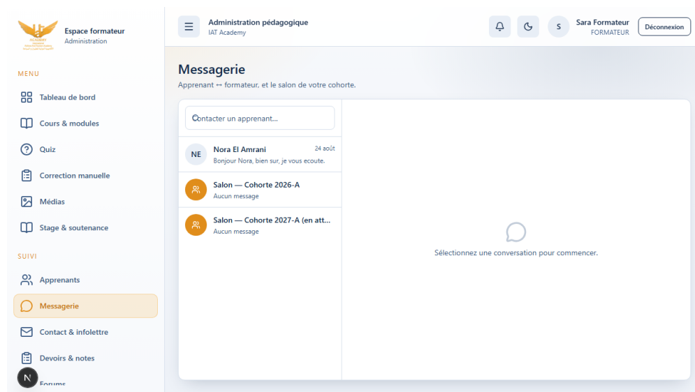
Figure 4.12. Salons de cohorte visibles dans la messagerie du formateur Descriptif : Avant ce correctif, un formateur ne voyait jamais les salons de ses cohortes dans sa propre messagerie, bien que le contrôle d'accès le lui permette déjà.
