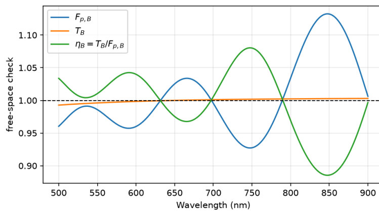
شکل ۹. خروجی مرجع فضای آزاد B : F_{p,B} ، T_B و \eta_B . خط‌چین مقدار ایده‌آل یک را نشان می‌دهد. نوسان منظم F_{p,B} با بازتاب ضعیف از PML یا درون‌یابی منبع سازگار است و \eta_B > 1 در 748 \text{ nm} غیرفیزیکی بودن آن را آشکار می‌کند.
