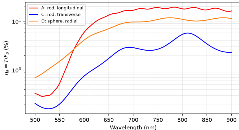
شکل ۳. بازده تابشی \eta_a = T/F_p حالت‌های A، C و D بر حسب طول‌موج (محور لگاریتمی). خط‌چین عمودی، طول‌موج قله‌ی پورسل حالت A است. در هر سه هندسه، گاف پنج‌نانومتری بازده را در تشدید به زیر ده درصد می‌راند.
