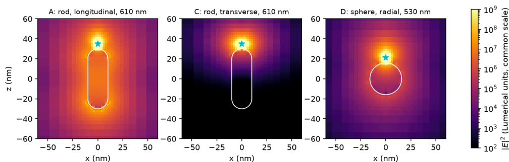
شکل ۸. نقشه‌ی لگاریتمی |E|^2 در صفحه‌ی xz برای A (نانومیل، طولی، 610 nm)، C (نانومیل، عرضی، 610 nm) و D (کره، شعاعی، 530 nm) با مقیاس رنگ مشترک. خط سفید مرز فلز و ستاره محل دوقطبی است؛ شعاع 3 nm حول منبع ماسک شده است.
