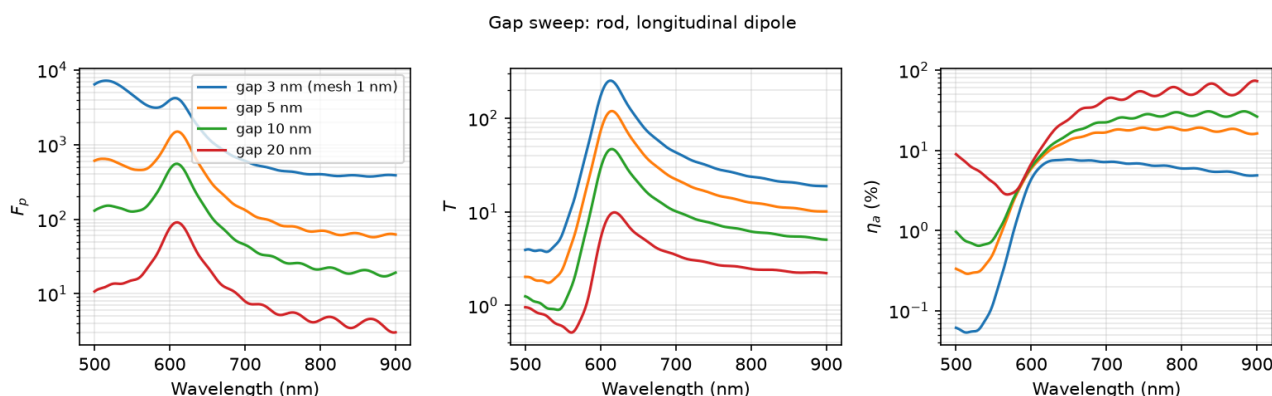
شکل ۵. پویش گاف برای نانومیل با دوقطبی طولی: F_p (چپ)، T (وسط) و \eta_a (راست) در گاف‌های 3 (مش 1 nm)، 5، 10 و 20 nm.
