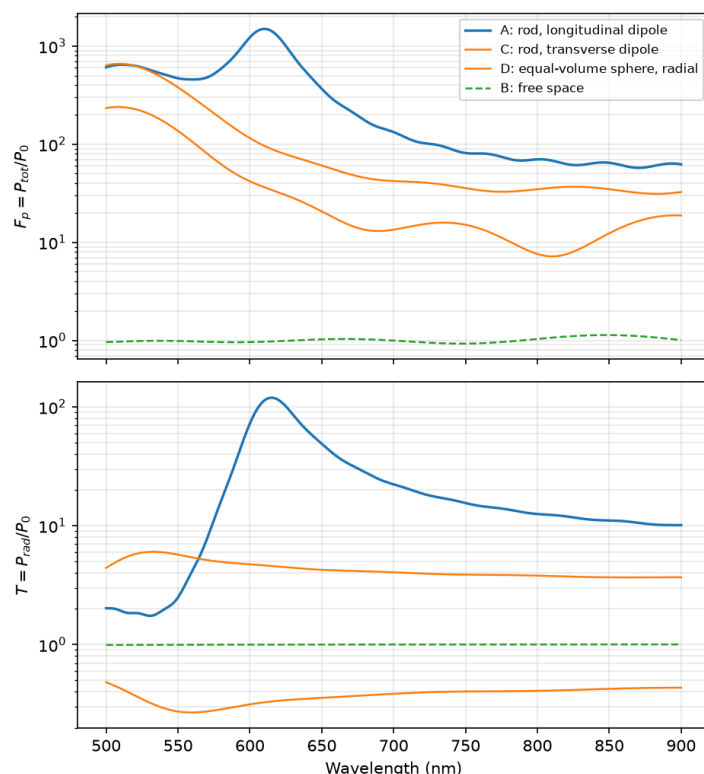
شکل ۲. فاکتور پورسل (بالا) و تقویت تابشی (پایین) حالت‌های A (نانومیل، طولی)، C (نانومیل، عرضی)، D (کره‌ای هم‌حجم، شعاعی) و مرجع فضای آزاد B، همه با تعریف خام و محور لگاریتمی، مستقیماً از فایل‌های ۲۰۱ نقطه‌ای.
