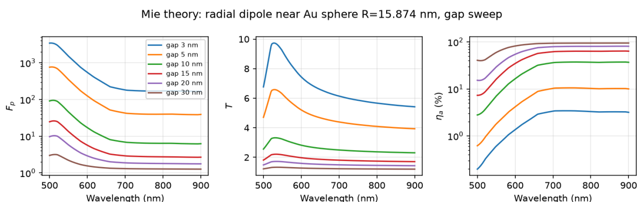
شکل ۶. پویش تحلیلی گاف (نظریه می) برای دوقطبی شعاعی کنار کره طلای R = 15.874 nm، برای مقایسه با شکل ۵.
