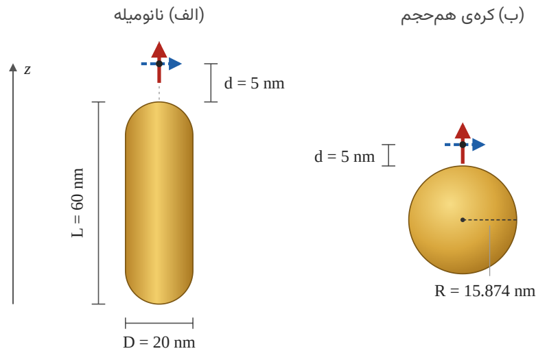
شکل ۱. طرح‌واره‌ی هندسه (گاف برای وضوح بزرگ‌تر از مقیاس رسم شده است). (الف) نانومیلیه‌ی طلای کلاهک‌دار با طول کل L و قطر D ؛ دوقطبی در فاصله‌ی d از رأس کلاهک بالایی روی محور z قرار دارد. (ب) کره‌ی طلای هم‌حجم برای حالت‌های D_{\perp} و D_{\parallel} . پیکان قرمز: دوقطبی در راستای z (حالت‌های A و D )؛ پیکان آبی خط‌چین: دوقطبی در راستای x (حالت‌های C و D_{\perp} ). کل ساختار درون جعبه‌ی شار مکعبی به ضلع 400 \text{ nm} و ناحیه‌ی FDTD به ضلع 600 \text{ nm} قرار دارد.
