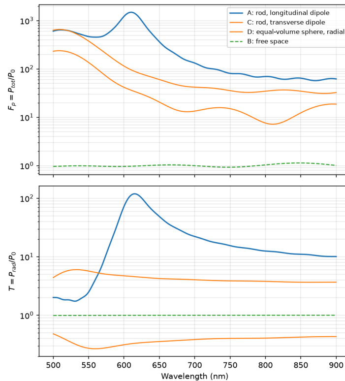
شکل ۳. فاکتور پورسل (بالا) و تقویت توان تابشی (پایین) حالت‌های A (نانومیله، طولی)، C (نانومیله، عرضی)، D (کره‌ی هم‌حجم، شعاعی) و مرجع فضای آزاد B، همه با تعریف خام و محور لگاریتمی، مستقیماً از فایل‌های ۲۰۱ نقطه‌ای.
