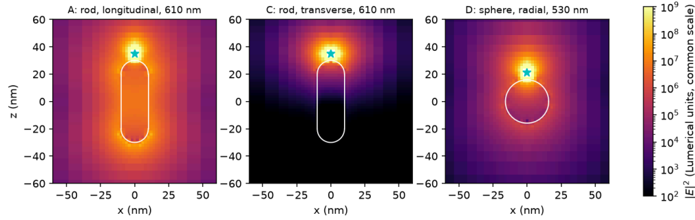
شکل ۹. نقشه‌ی لگاریتمی |E|^2 در صفحه‌ی xz برای A (نانومیله، طولی، 610 nm)، C (نانومیله، عرضی، 610 nm) و D (کره، شعاعی، 530 nm) با مقیاس رنگ مشترک. خط سفید مرز فلز و ستاره محل دوقطبی است؛ شعاع 3 nm حول منبع ماسک شده است.
