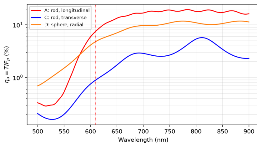
شکل ۴. بازده تابشی \eta_a = T/F_p حالت‌های C، A، و D بر حسب طول‌موج (محور لگاریتمی). خط‌چین عمودی، طول‌موج قله‌ی پورسل حالت A است. در هر سه هندسه، گاف پنج‌نانومتری بازده را در تشدید به زیر ده درصد می‌راند.
