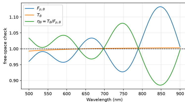
شکل ۱۰. خروجی مرجع فضای آزاد B: F_{p,B} ، T_B و \eta_B . خط چین مقدار ایده‌آل یک را نشان می‌دهد. نوسان منظم F_{p,B} با بازتاب ضعیف از PML یا درون‌یابی منبع سازگار است و \eta_B > 1 در 748 \text{ nm} غیرفیزیکی بودن آن را آشکار می‌کند.
