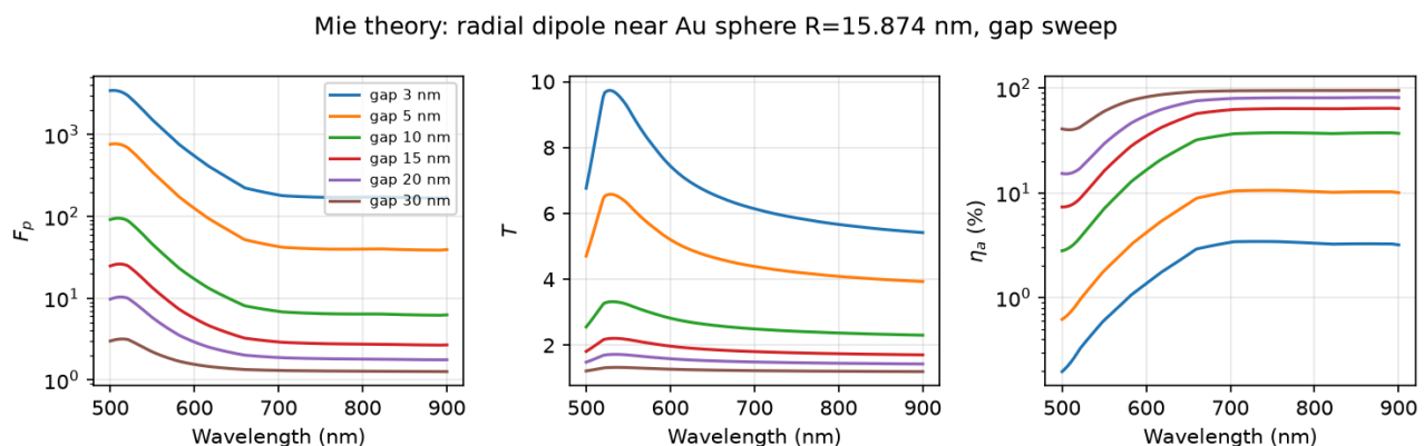
شکل ۷. پویش تحلیلی گاف (نظریه‌ی می) برای دوقطبی شعاعی کنار کره‌ی طلای R = 15.874 \text{ nm} ، برای مقایسه با شکل ۶.
