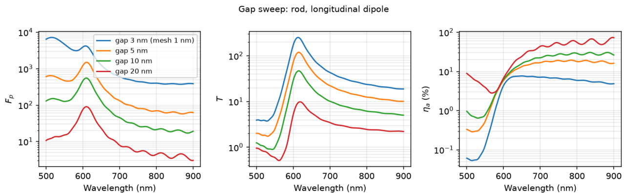
شکل ۶. پویش گاف برای نانومیله با دوقطبی طولی: F_p (چپ)، T (وسط) و \eta_a (راست) در گاف‌های 3 (مش 1 nm)، 5، 10 و 20 nm.
