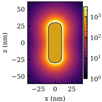
LDOS \rho/\rho_0 , 608 nm
