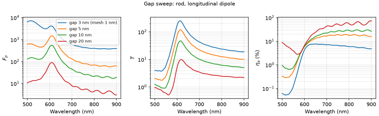
شکل ۷. پویش گاف برای نانومیله با دوقطبی طولی: F_p (چپ)، T (وسط) و \eta_a (راست) در گاف‌های 3 (مش 1 nm)، 5، 10 و 20 nm.
