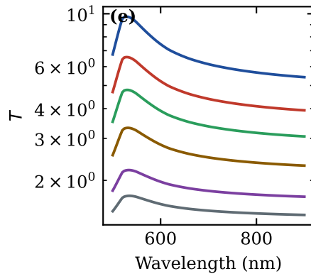
sphere, radial (Mie)
