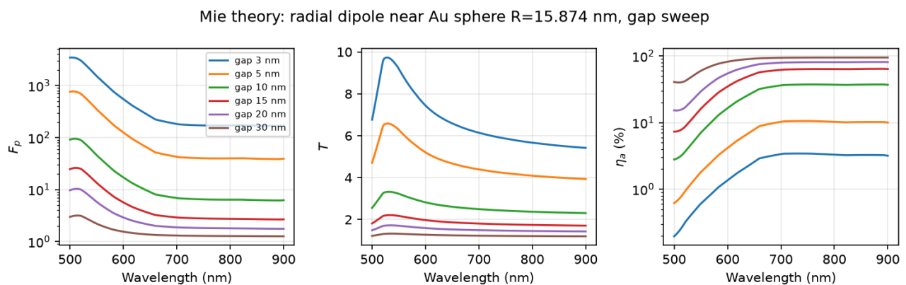
شکل ۷. پویش تحلیلی گاف (نظریه‌ی می) برای دوقطبی شعاعی کنار کره‌ی طلای R = 15.874 nm، برای مقایسه با شکل ۶.
