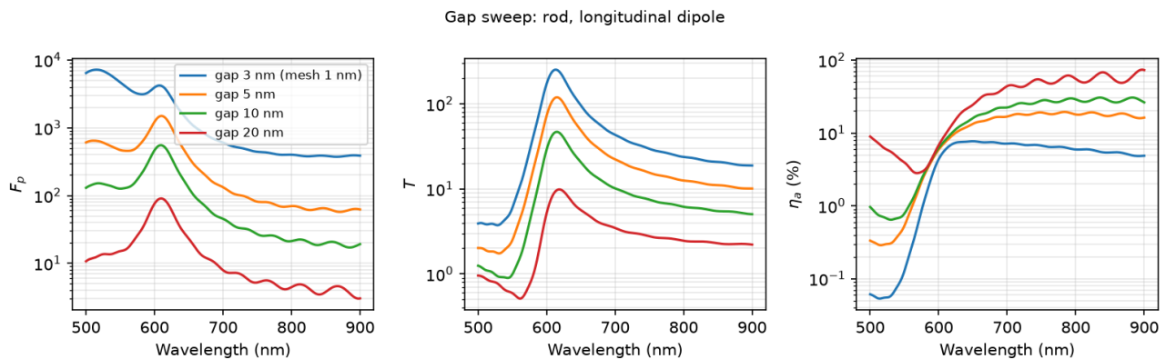
شکل ۶. پویش گاف برای نانومیله با دوقطبی طولی: F_p (چپ)، T (وسط) و \eta_a (راست) در گاف‌های 3 (مش 1 nm)، 5، 10 و 20 nm.
