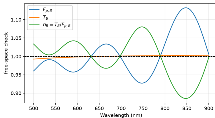
شکل ۱۰. خروجی مرجع فضای آزاد B: F_{p,B} ، T_B و \eta_B . خط‌چین مقدار ایده‌آل یک را نشان می‌دهد. نوسان منظم F_{p,B} با بازتاب ضعیف از PML یا درون‌یابی منبع سازگار است و \eta_B > 1 در 748 nm غیرفیزیکی بودن آن را آشکار می‌کند.
