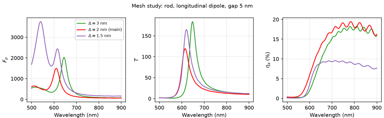
شکل ۸. همگرایی مش برای نانومیله با دوقطبی طولی در گاف 5 \text{ nm} : F_p (چپ)، T (وسط) و \eta_a (راست) برای مش موضعی 3، 2 و 1.5 \text{ nm} . مکان قله‌ی تابشی و بازده در آن پایدارند؛ ارتفاع قله‌ها به قرارگیری زیرسلولی چشمه حساس است.
