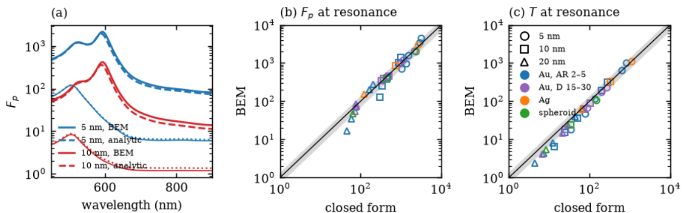
(a) حل نیمه‌تحلیلی در برابر BEM برای بیضی‌گون. (b) و (c) F_p و T در تشدید: BEM در برابر فرمول بسته برای ۳۰ پیکرنندی.
