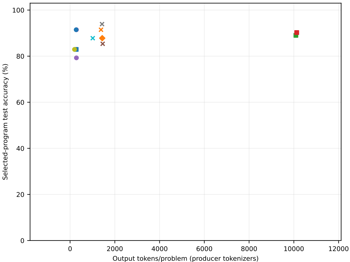
humanevalplus
