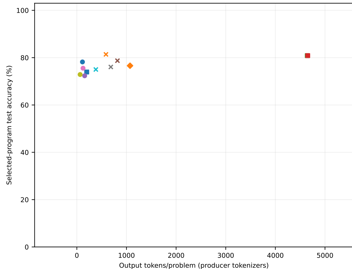
mbppplus
