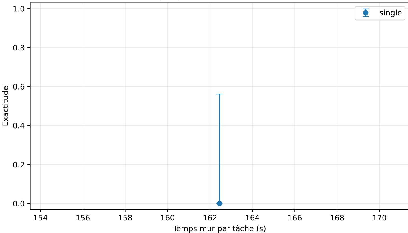
Pilote descriptif présélectionné, n=3 ; Wilson 95 %
