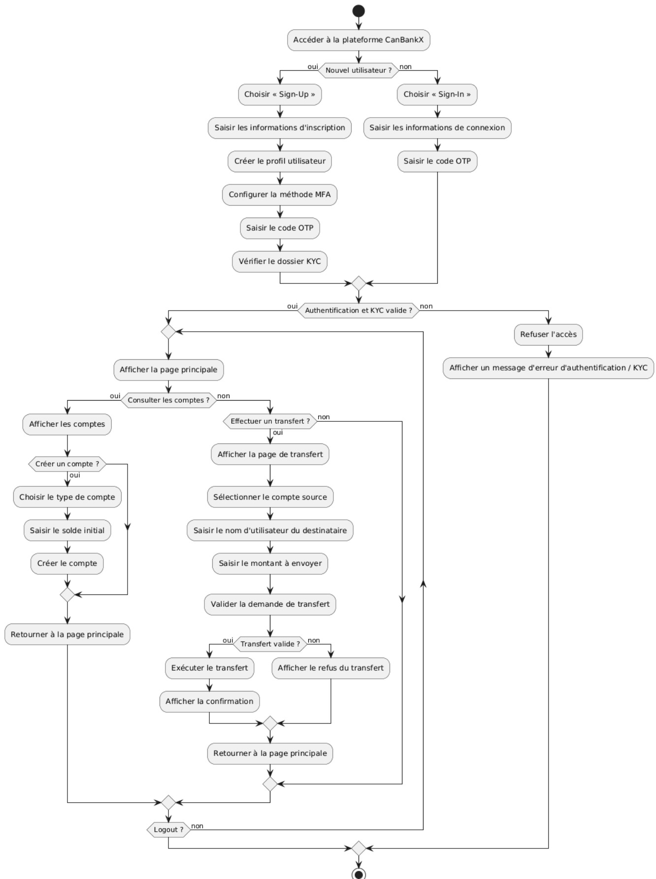
CanBankX - Diagramme d'activité (Portée et contexte)
