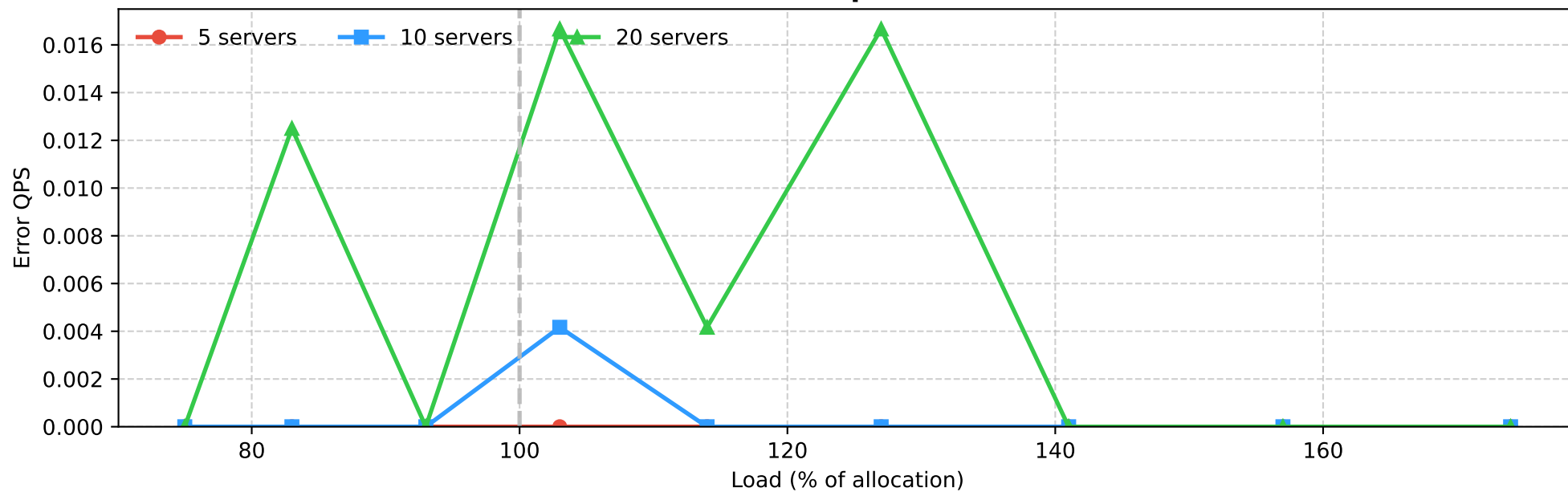
Prequal
