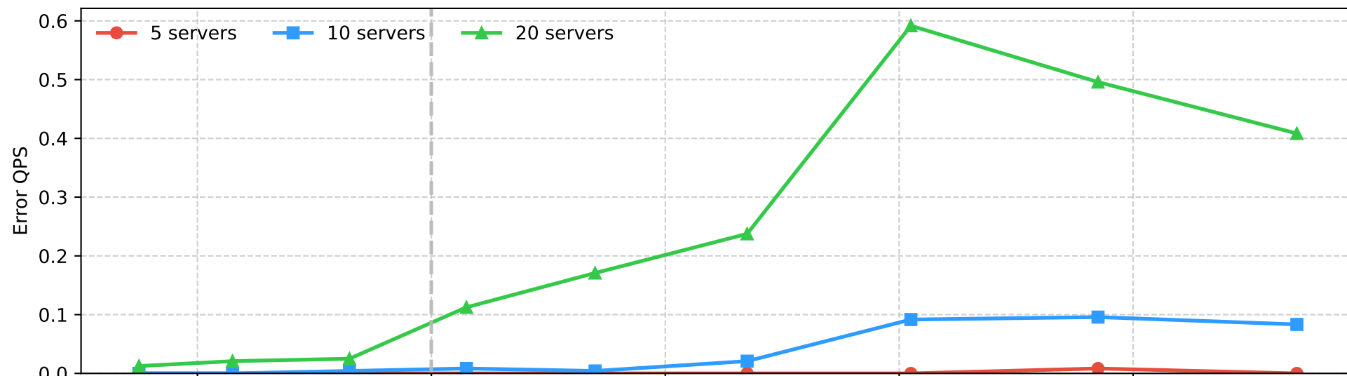
WRR
