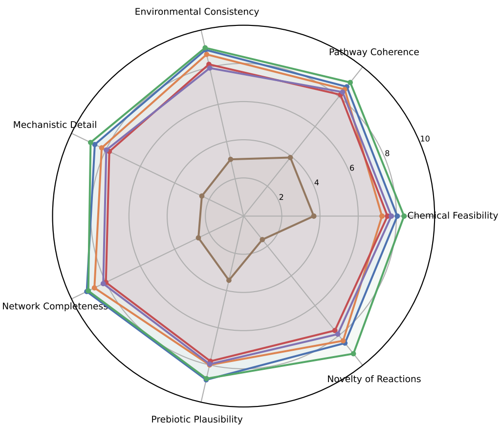
claude_opus4.6
