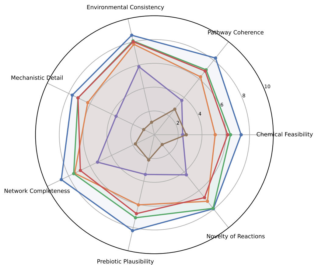
gpt41
