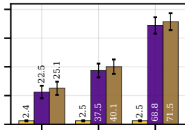
llama.cpp (F16)
