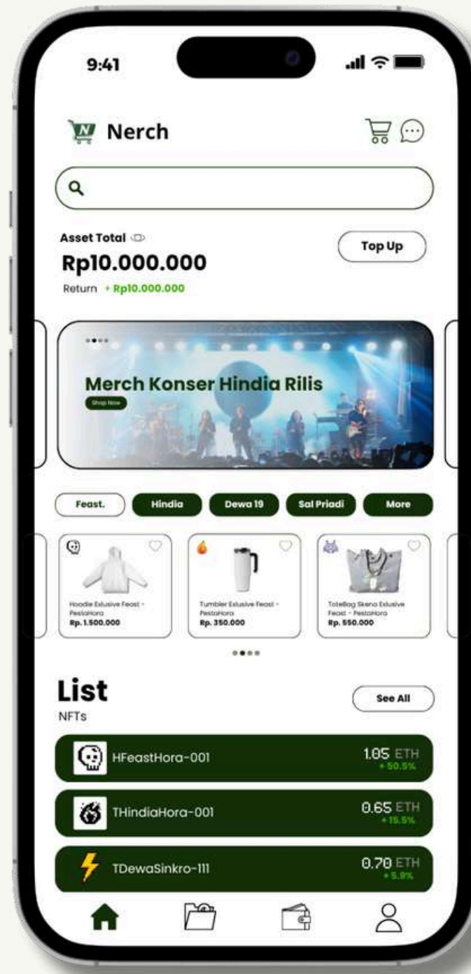
Dashboard utama
