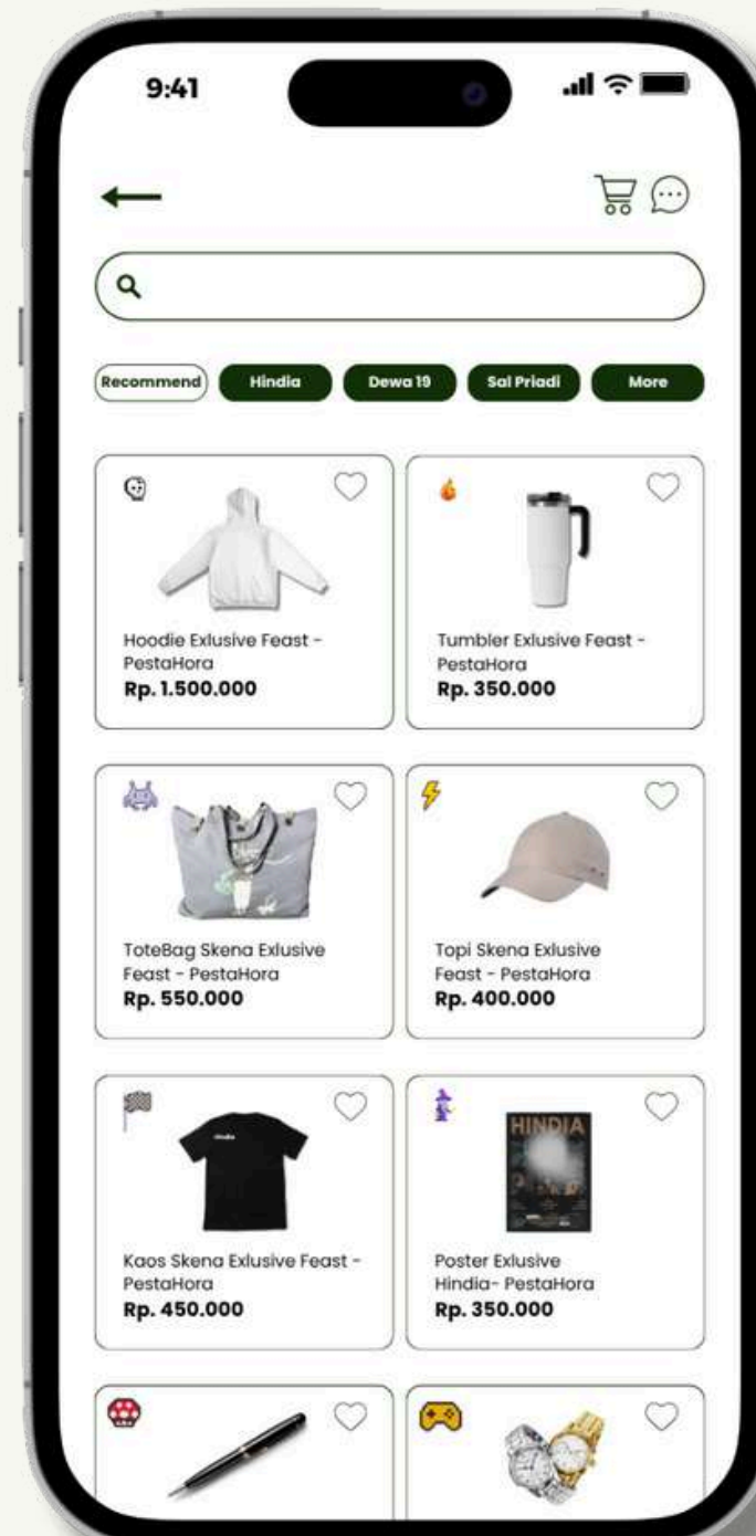
Katalog Produk
