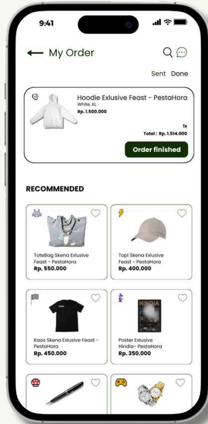
Sistem Escrow
