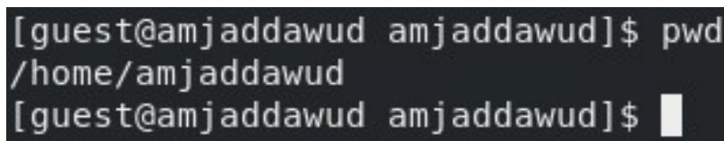
Рисунок 3.5: Комманда pwd
