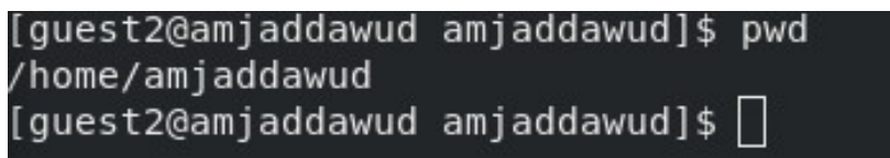
Рисунок 3.6: Комманда pwd
