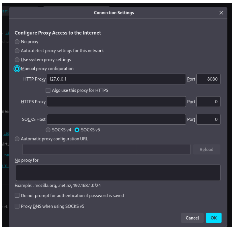
Рисунок 3.4: Настройки сервера
