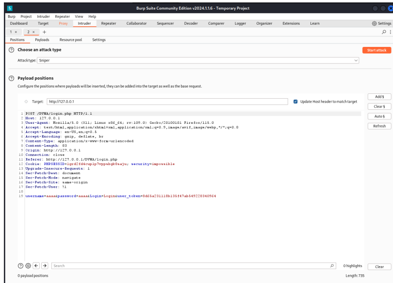
Рисунок 3.13: Вкладка Intruder
