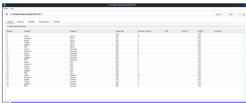
Рисунок 3.17: Запуск атаки
