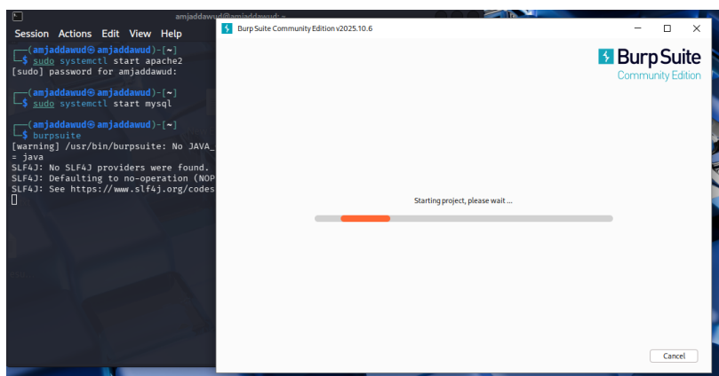
Рисунок 3.2: Запуск приложения
