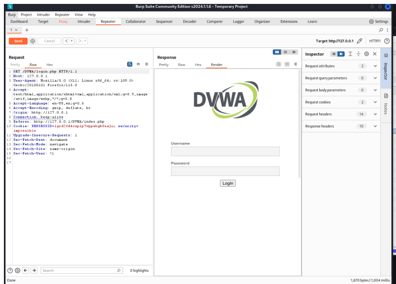
Рисунок 3.24: Полученная страница
