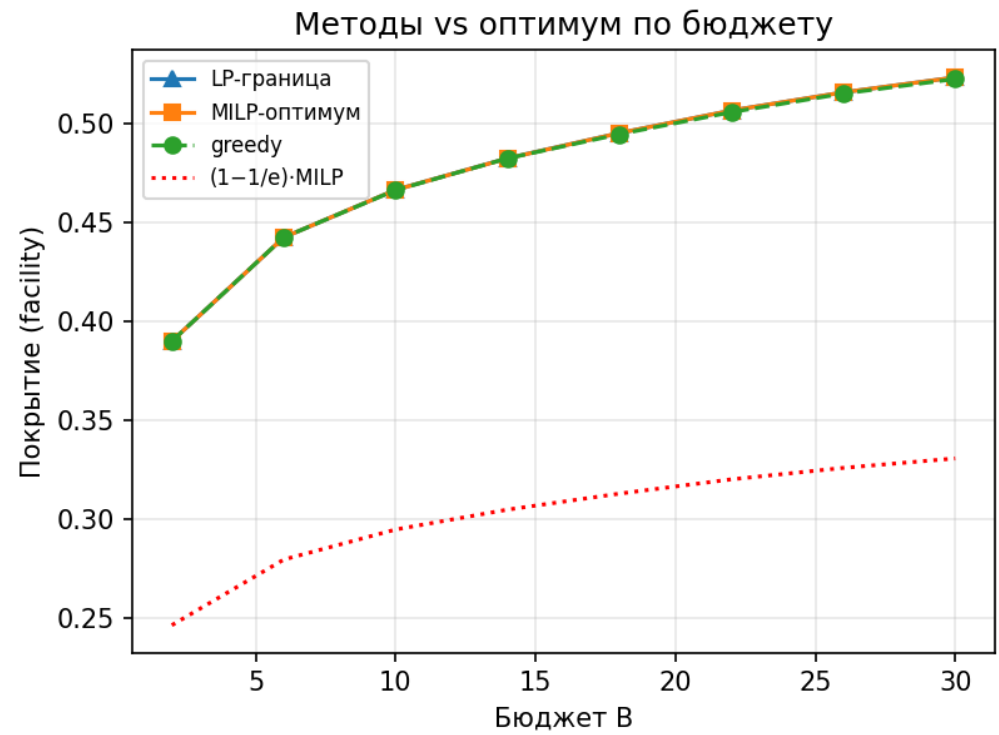
Сравнение методов оптимизации по бюджету
