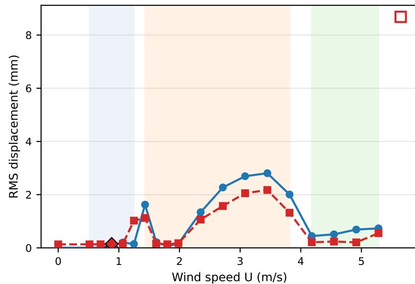
(d) Torsion RMS
