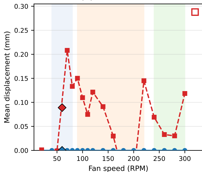
(d) Torsion Mean
