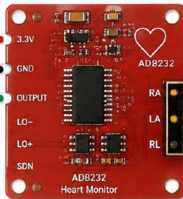
MÓDULO AD8232
