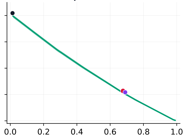
DeepSeek V3.2
