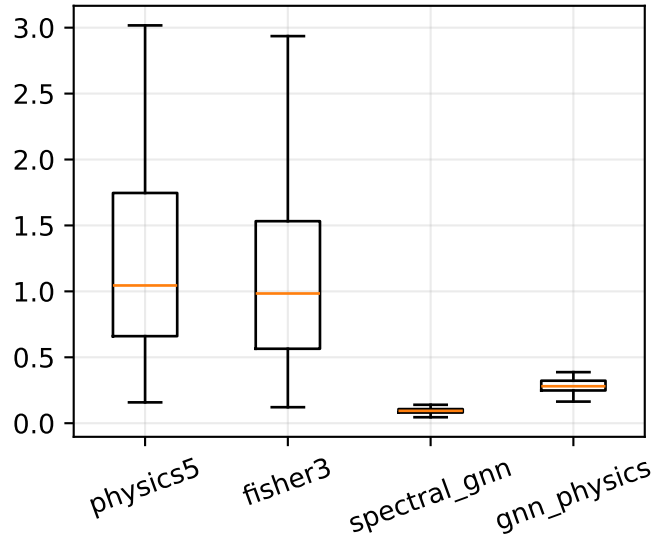
5-D parameter RMSE
