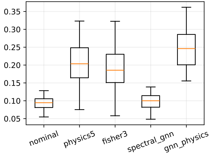
5-D parameter RMSE
