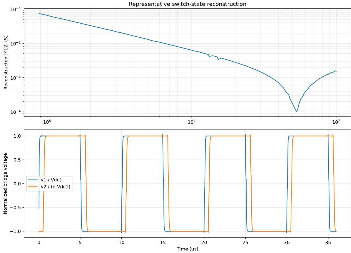
图 19: 代表性多端口 Y_{12} 重构与含死区、有限边沿的原副边开关状态电压。
