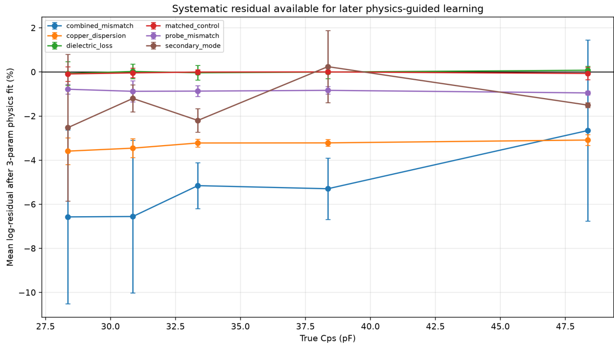
图 16: 三参数物理拟合后的对数残差随真实 C_{ps} 的变化。组合失配与铜阻/漏感频变呈现稳定负偏差，但组合场景在部分电容状态下方差较大，提示后续模型应同时输出不确定度。
