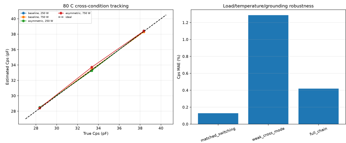
图 18: 开关状态 DAB 多工况 C_{ps} 跟踪与三种前向层级误差。完整链路在未改变反演模型的情况下仍保持亚百分比级跟踪。
