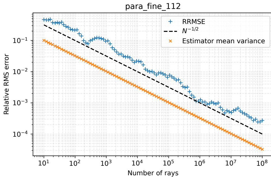
FIGURE 2.1 – Facteurs de vue estimés par E2T pour un parallélépipède
