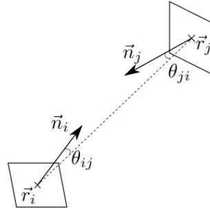
FIGURE 1.3 – Illustration des notations géométriques introduites à l'Eq ??
