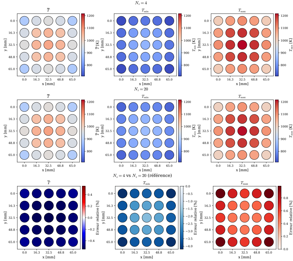
FIGURE .9 – Champs de température pour \bar{T} = 981,4 K : N_z = 4 (haut), N_z = 20 (milieu) et différence entre les deux champs (bas).
