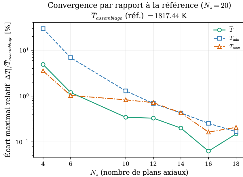
FIGURE 6.7 – Écart relatif des températures minimale, maximale et moyenne en fonction de N_z , par rapport à la référence N_z = 20 , pour le niveau de puissance le plus élevé.
