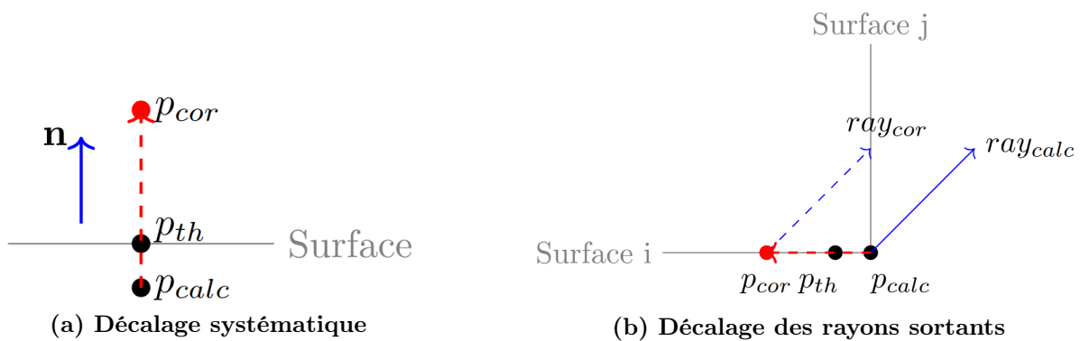
FIGURE 3.3 – Illustration en 2D des décalages nécessaires pour corriger l'imprécision flottante.
