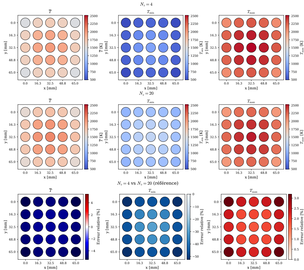
FIGURE 6.6 – Champs de température pour le niveau de puissance le plus élevé : N_z = 4 (haut), N_z = 20 (milieu) et différence entre les deux champs (bas).
