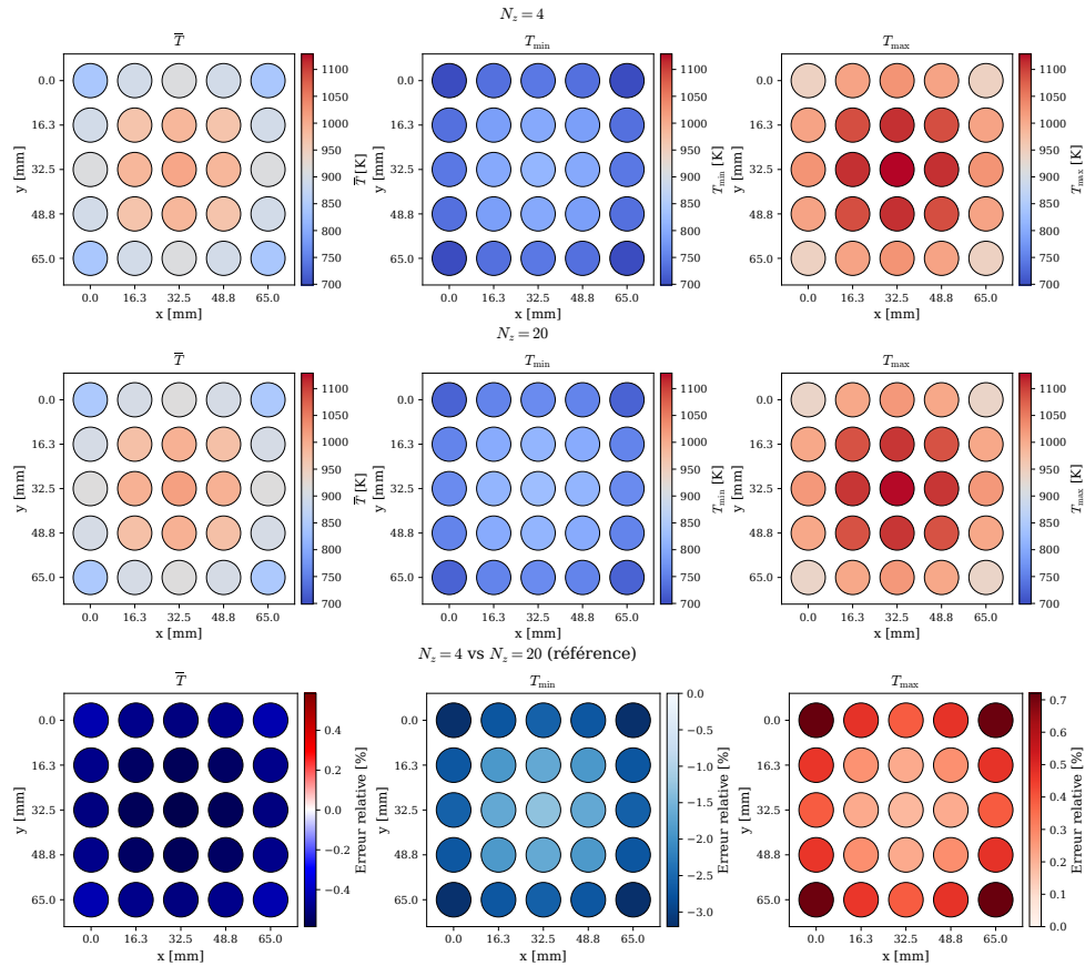
FIGURE 6.4 – Champs de température pour \overline{T} = 925,7 K : N_z = 4 (haut), N_z = 20 (milieu) et différence entre les deux champs (bas).
