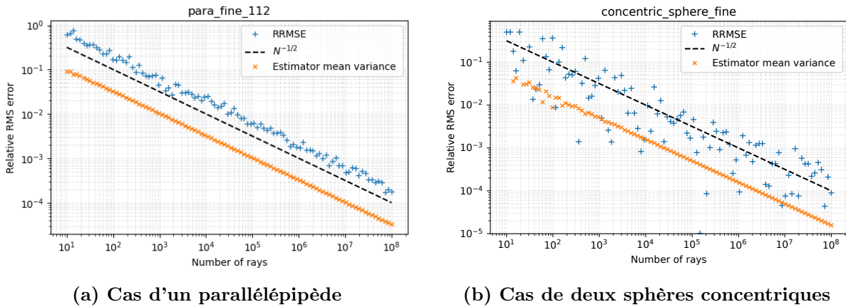
FIGURE 4.1 – Convergence des facteurs de vue pour deux géométries tridimensionnelles.
