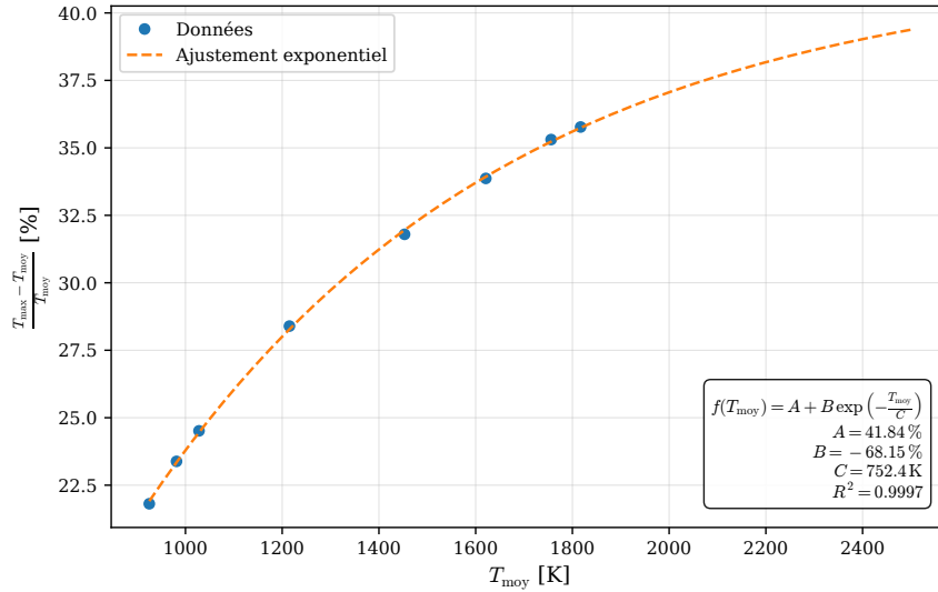
FIGURE 6.8 – Modélisation de l'écart de la température maximale par rapport à la température moyenne.
