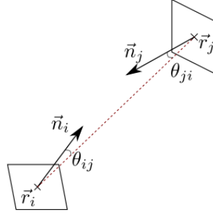
FIGURE 3 – Illustration des notations géométriques introduites à l'Eq ??
