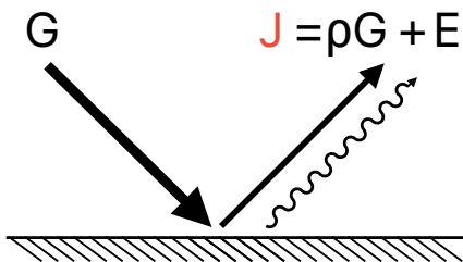
FIGURE 1 – Échanges radiatifs considérés dans le problème
