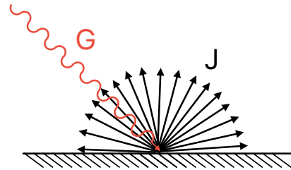
FIGURE 2 – Illustration de l'hypothèse de réflexion et émission diffuse
