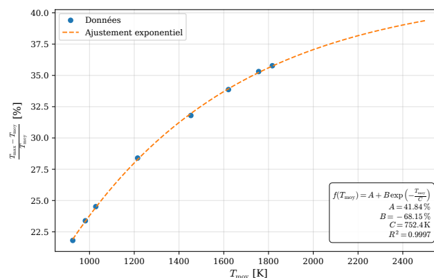
FIGURE 6.8 – Modèle de l'écart de la température maximale par rapport à la température moyenne.
