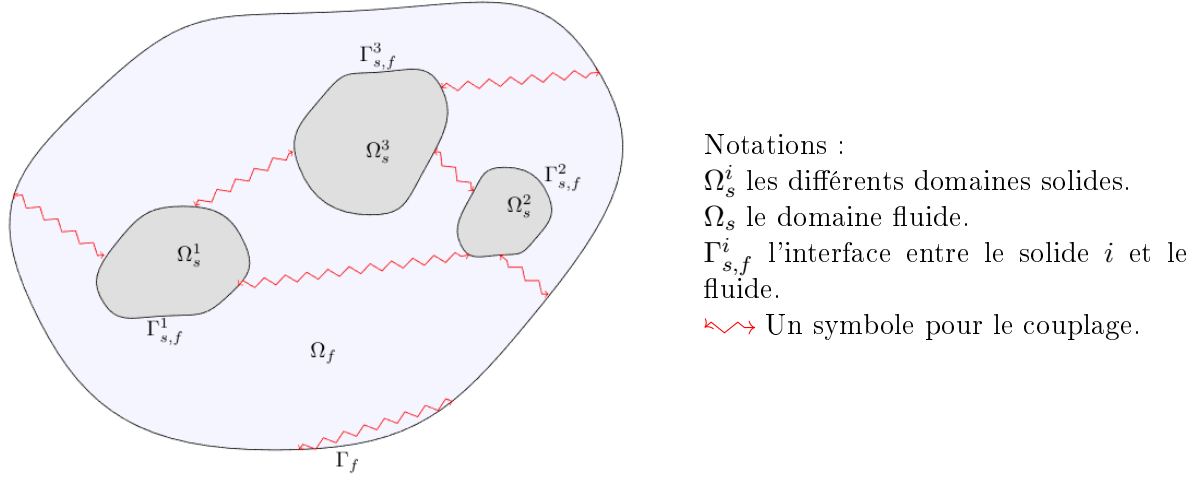
FIGURE 5.1 – Schéma typique d'un problème de couplage conduction-rayonnement en milieu transparent
