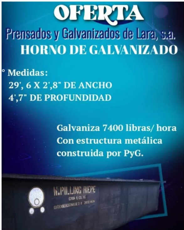
Horno de Galvanizado — Placa W. Pilling Riepe Identificación del fabricante alemán en el horno de galvanizado.
